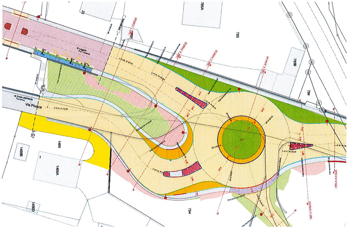
Estratto progetto cantonale nuova rotonda
