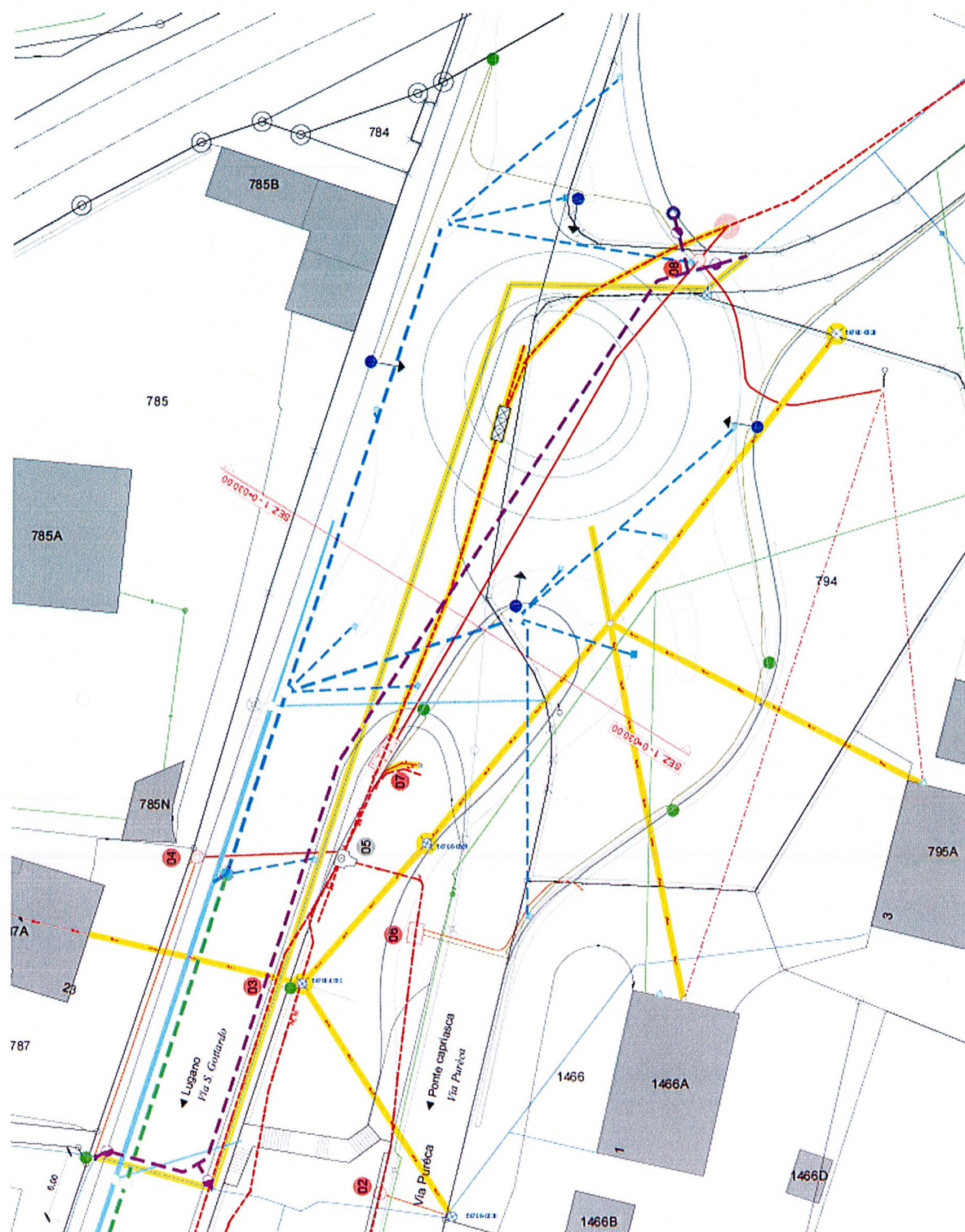
Planimetria delle infrastrutture
