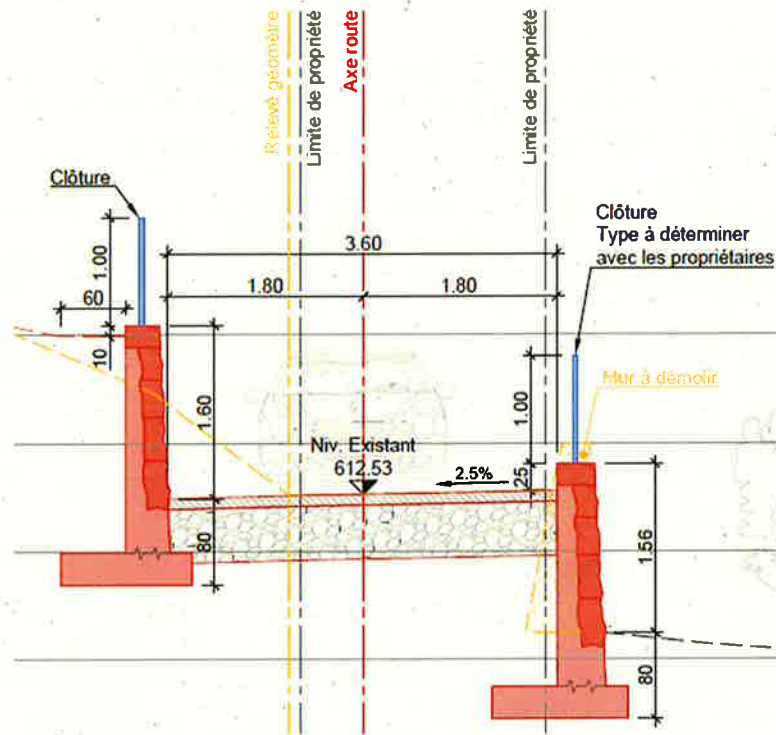
Coupe type des travaux
