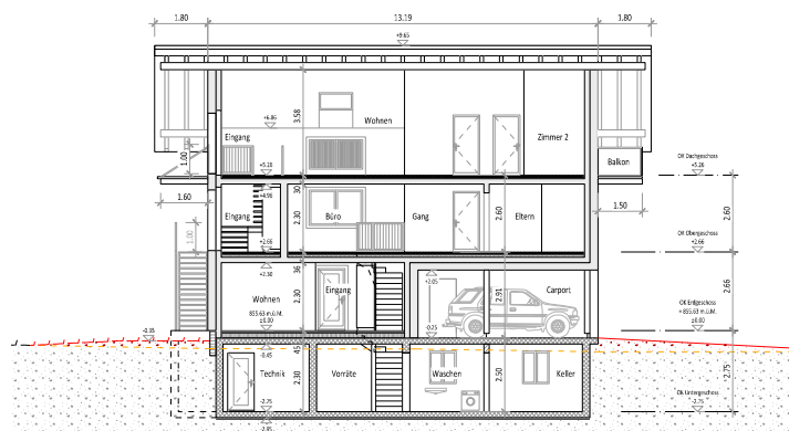
Längsschnitt A-A
