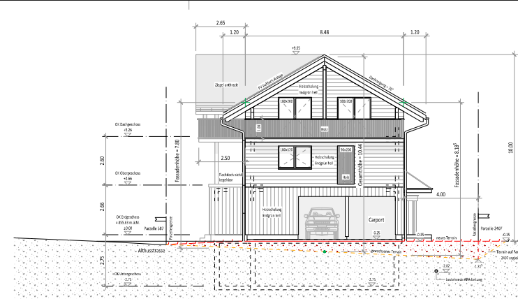
Südostfassade
