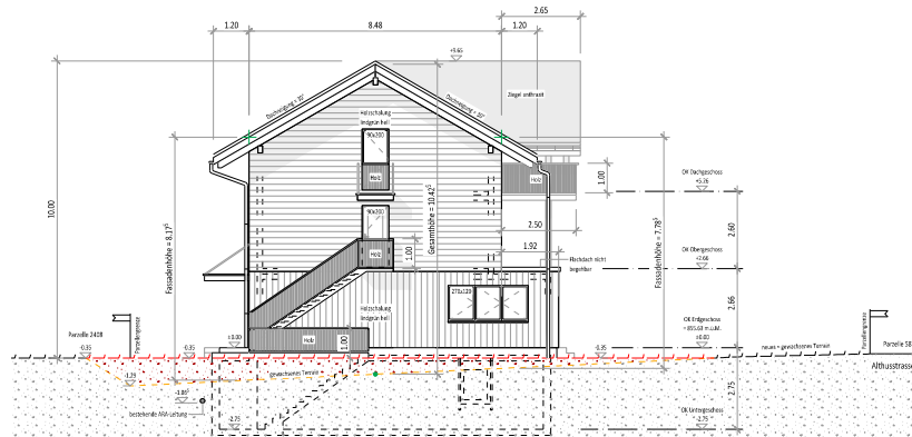
Nordwestfassade
