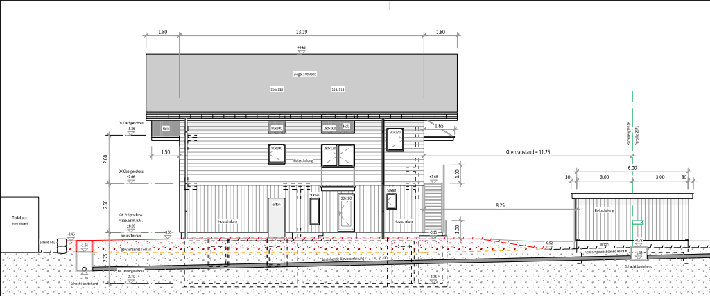
Nordostfassade
