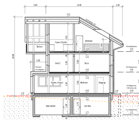
Querschnitt B-B
