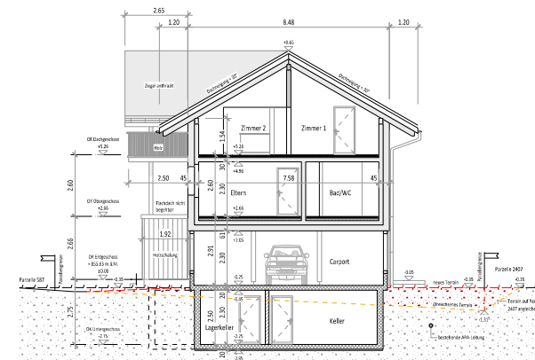
Querschnitt C-C
