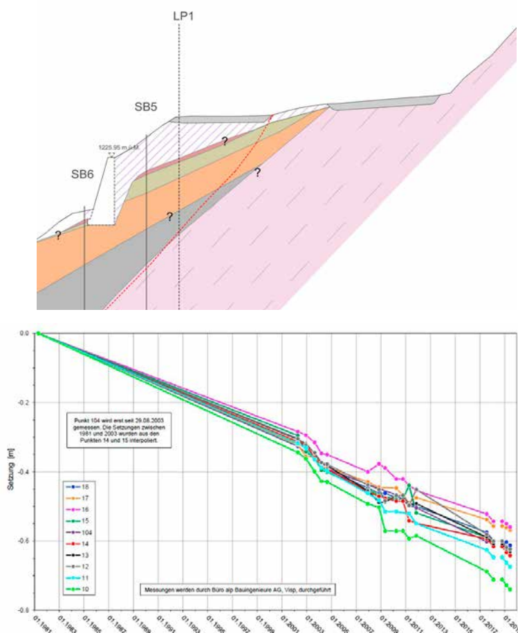
Schichtverlauf und gemessene Setzungen der bestehenden Stützmauer
