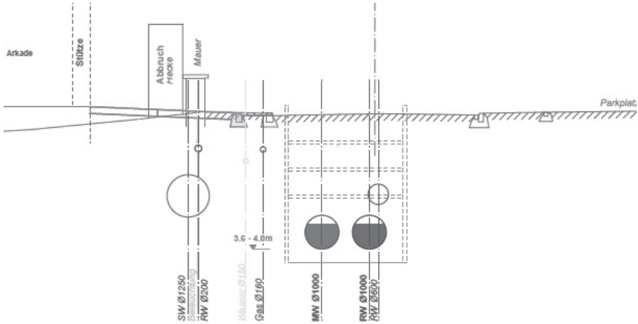
Grabenprofil Bahnhofstrasse
