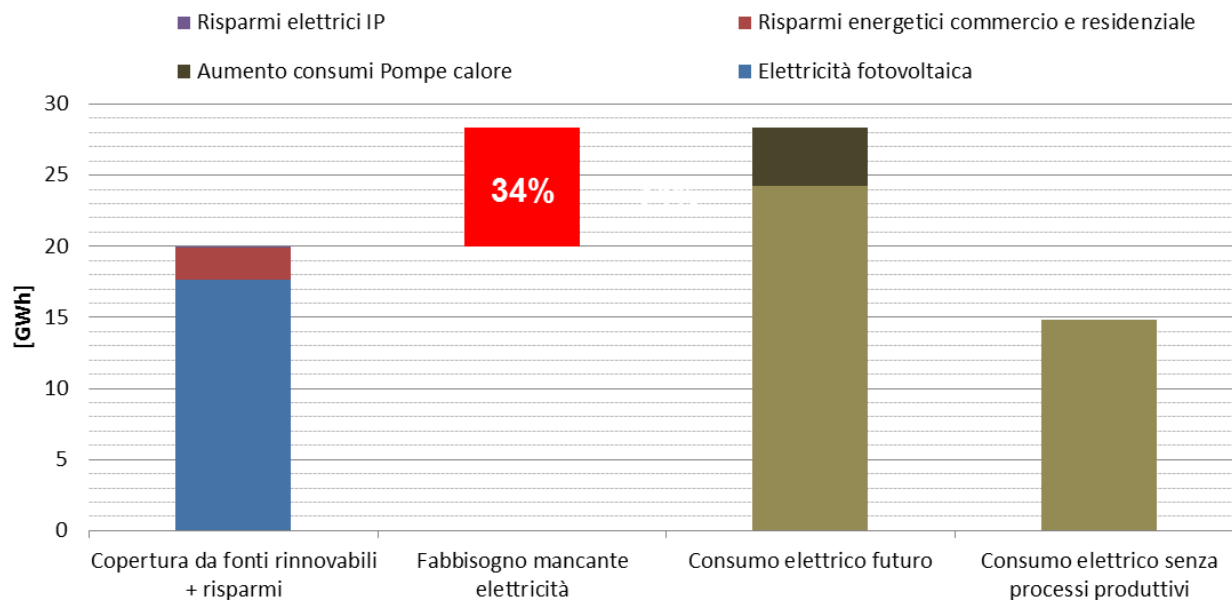
Figura 2: confronto tra i potenziali del territorio comunale di produzione di energia elettrica da fonti rinnovabili e consumi elettrici futuri calcolati sulla base dei potenziali di risparmio elettrico e degli aumenti prodotti dalle pompe di calore. Il grafico indica anche il gap energetico da colmare con l'importazione.
