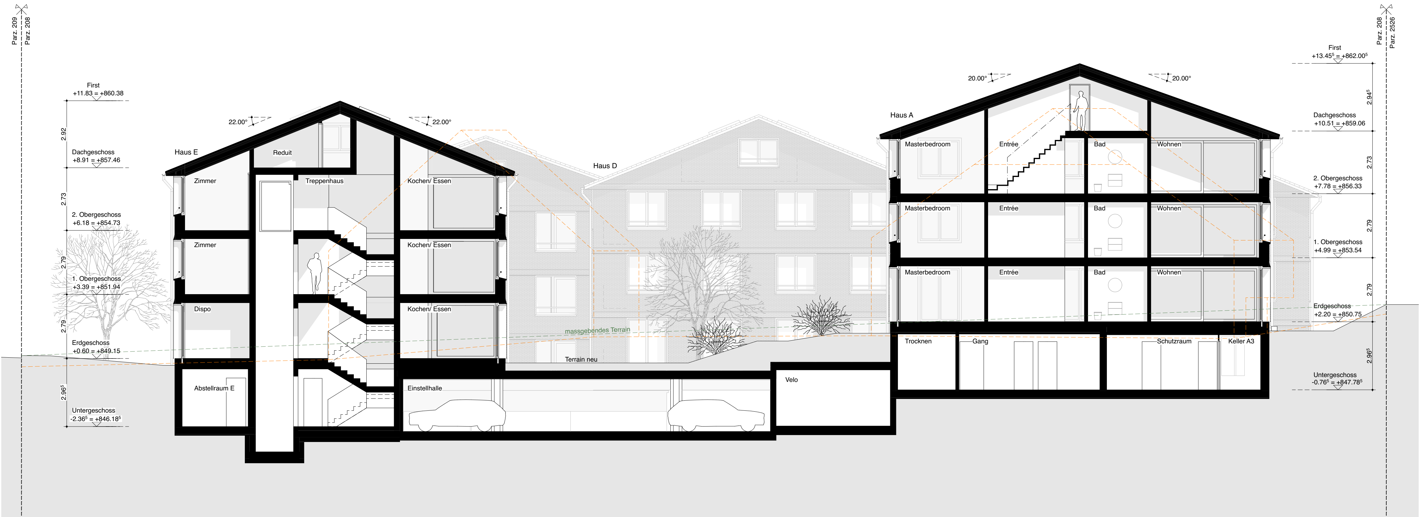
SCHNITT A-A
