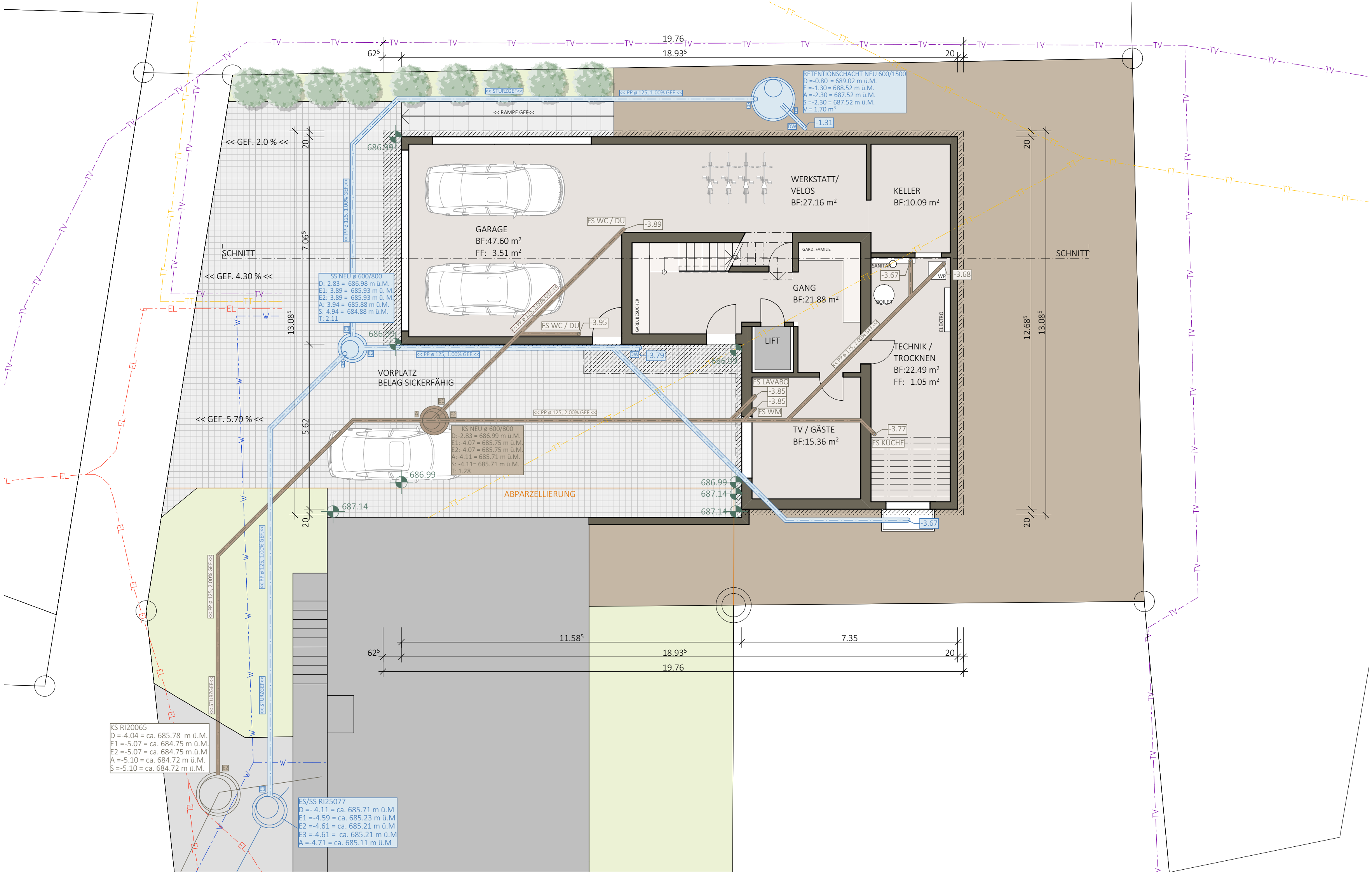
GRUNDRISS UNTERGESCHOSS + KANALISATION
