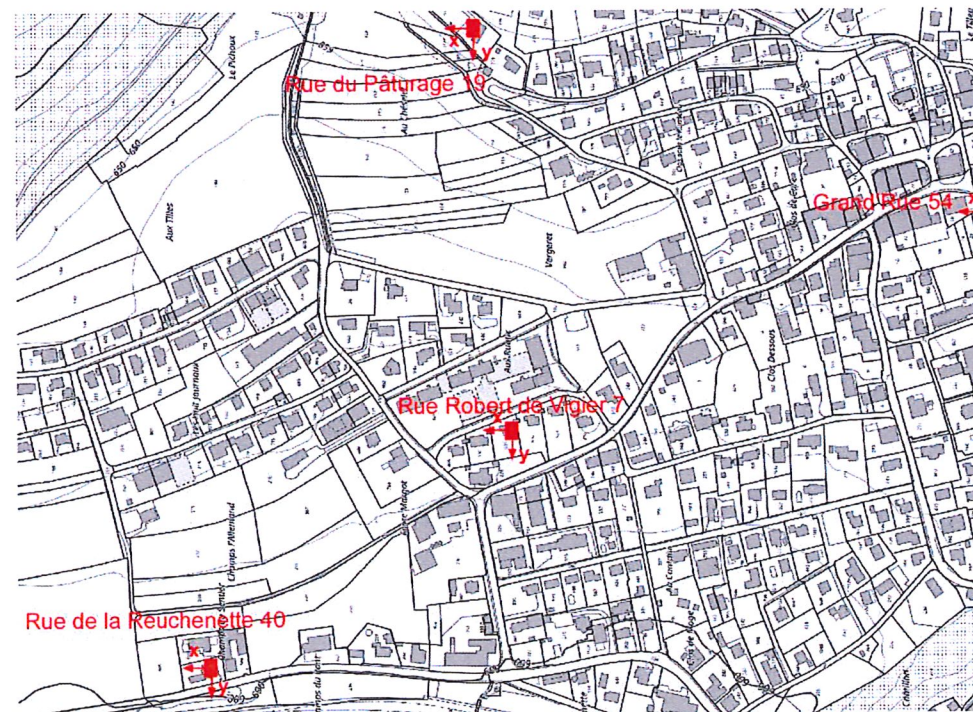
Fig. 01: Position des capteurs de vibrations avec orientation des composantes horizontales (x,y)
