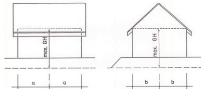
Gebäudehöhe (Art. 34)
