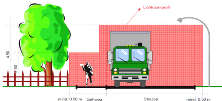
Das Lichtraumprofil
