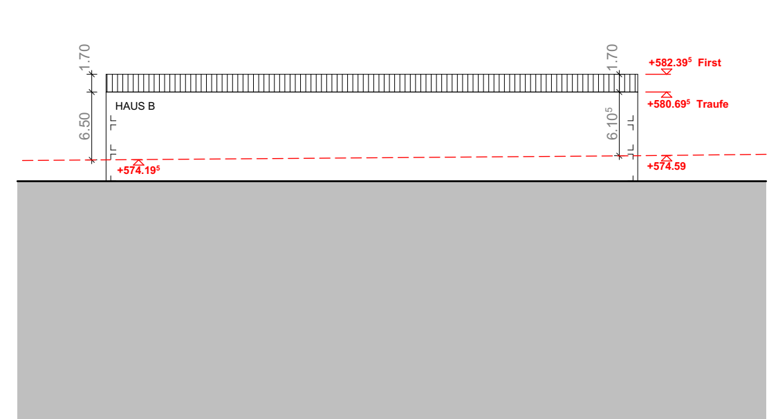
Haus B Ostseite
