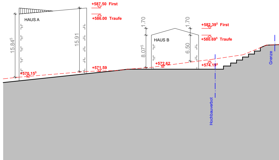
Haus A und B Südseite
