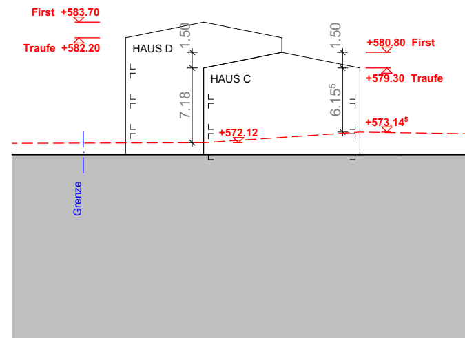
Haus C und D Ostseite
