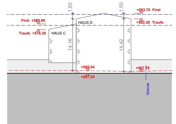
Haus C und D Westseite
