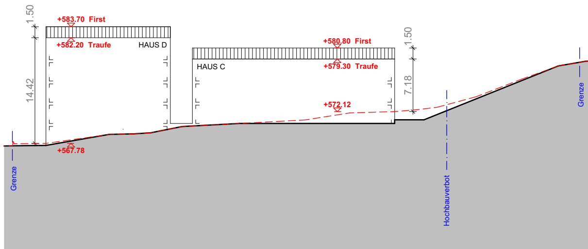
Haus C und D Südseite
