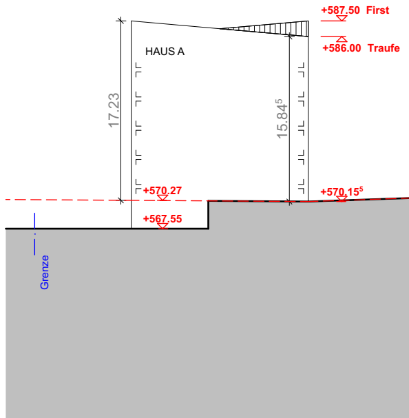
Haus A Westseite
