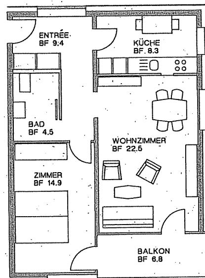
Wohnungstyp 2 Zimmer Süd BF 59.6 m 2 1.-4. Obergeschoss
