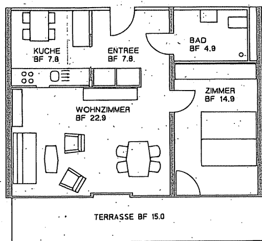
Wohnungstyp 2 Zimmer BF 58.3 m 2 Attikageschoss
