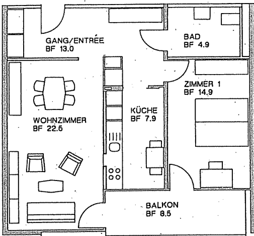
Wohnungstyp 2 Zimmer BF 63.2 m 2 1.-4. Obergeschoss
