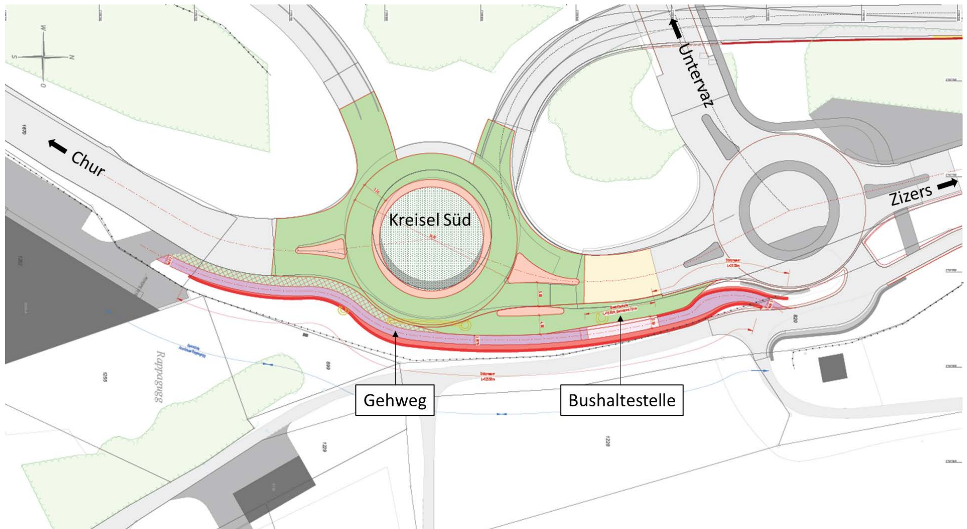
Situationsplan mit geplantem Gehweg und Bushaltestelle
