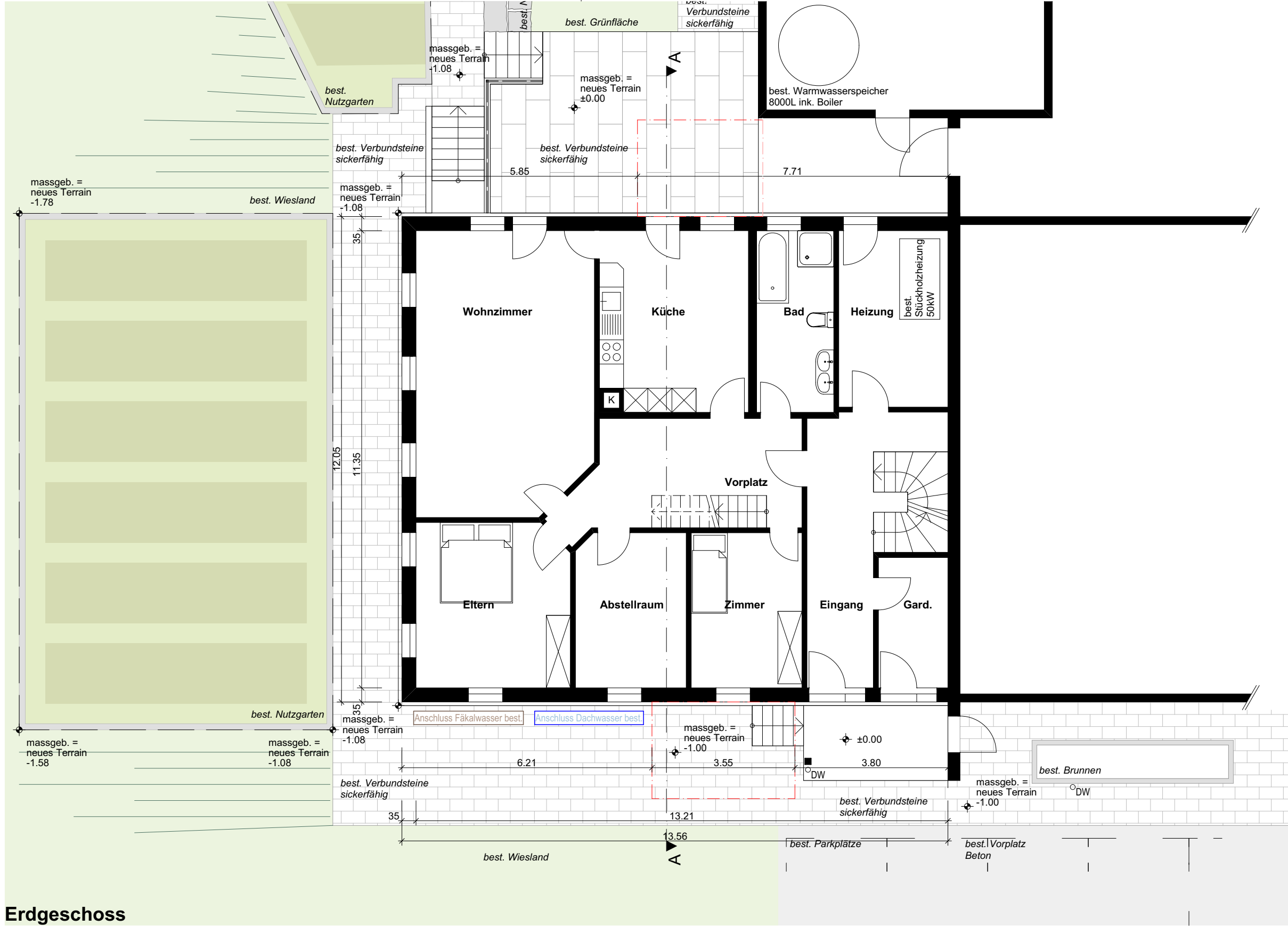
Erdgeschoss
