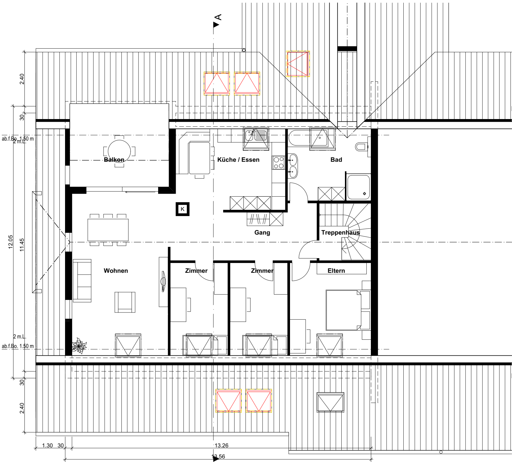
Dachgeschoss
