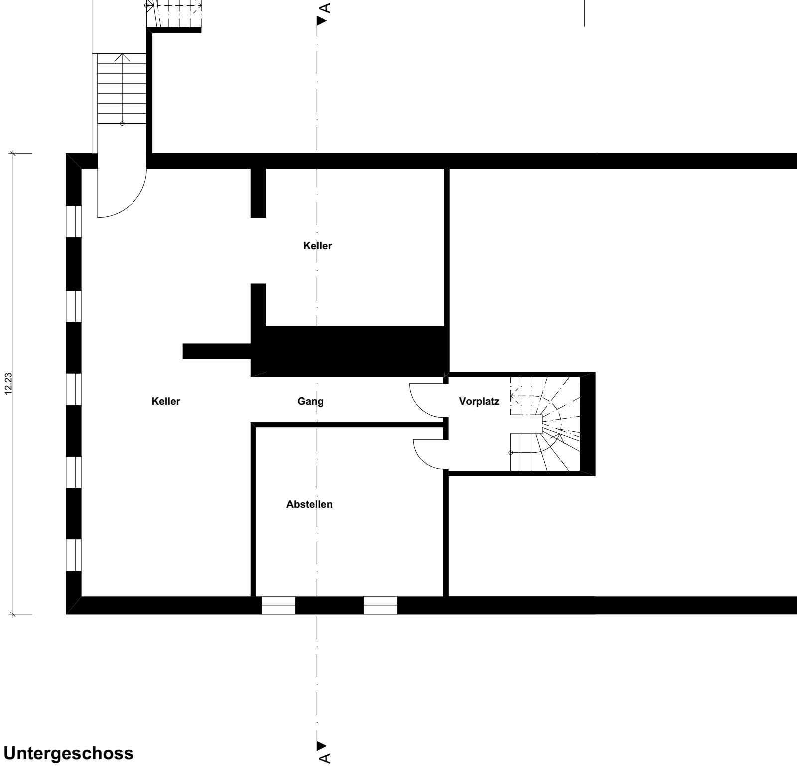
Untergeschoss
