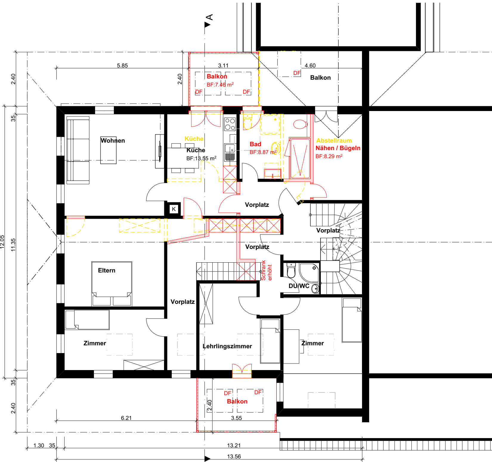
Obergeschoss
