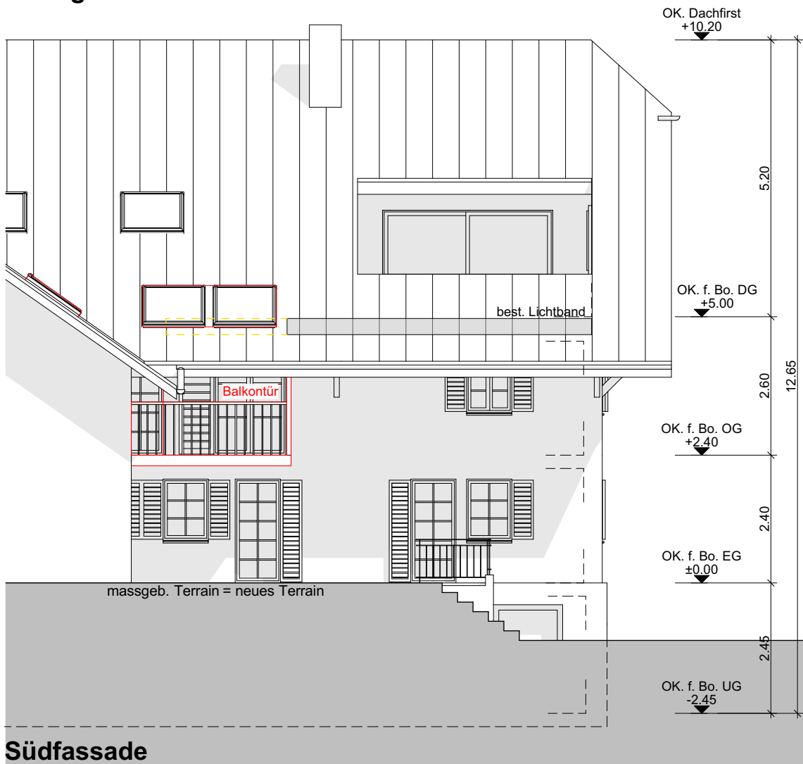
Südfassade
