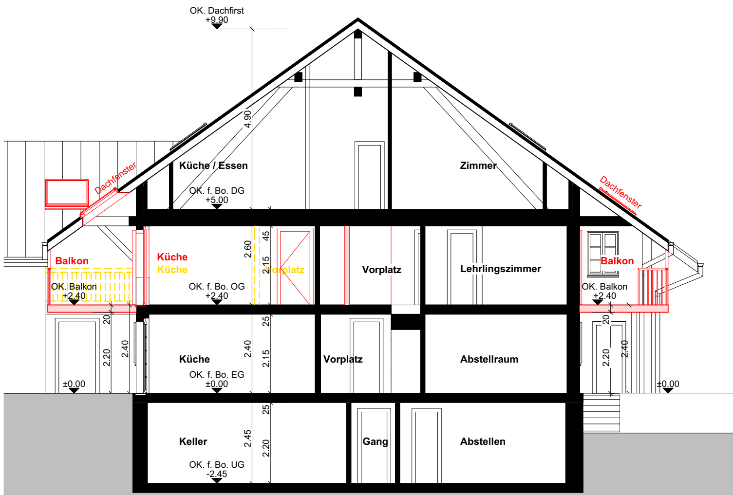
Schnitt A-A
