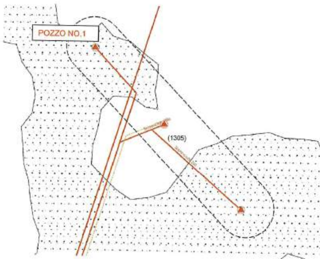
Dettaglio 3 pozzi AIAP:
