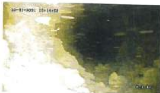
6, 00:08:48, 24.50m Grossa formazione di depositi duri nella giunzione, da ore 12 a ore 12
