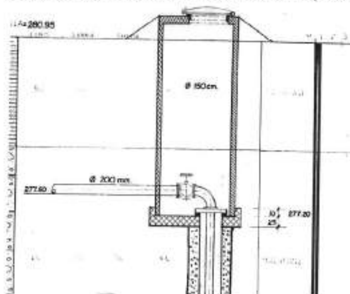
Figura 2 Estratto dalla stratigrafia del sondaggio Pozzo 1 fornita da UT Caslano (Allegato A)
