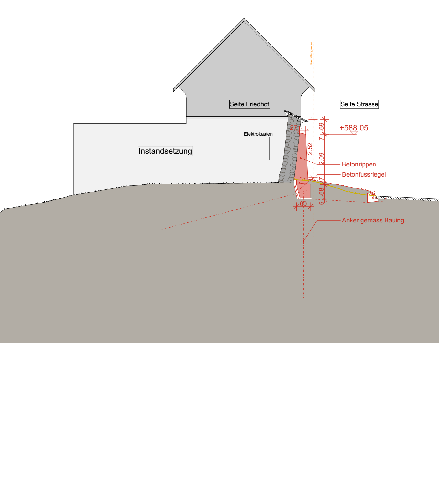
Schnitt A
