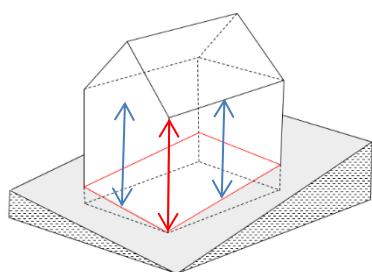
Abb. 19 Messweise Gebäudehöhe (bisher) und Fassadenhöhe traufseitig (neu)
