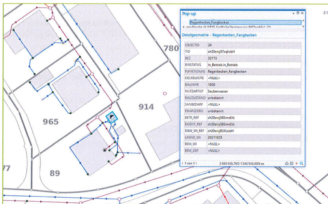
Abbildung 5 - Im Bereich der privaten Liegenschaftsentwässerung wird eher ein Versickerungsschacht anstelle des Fangbeckens erwartet.
