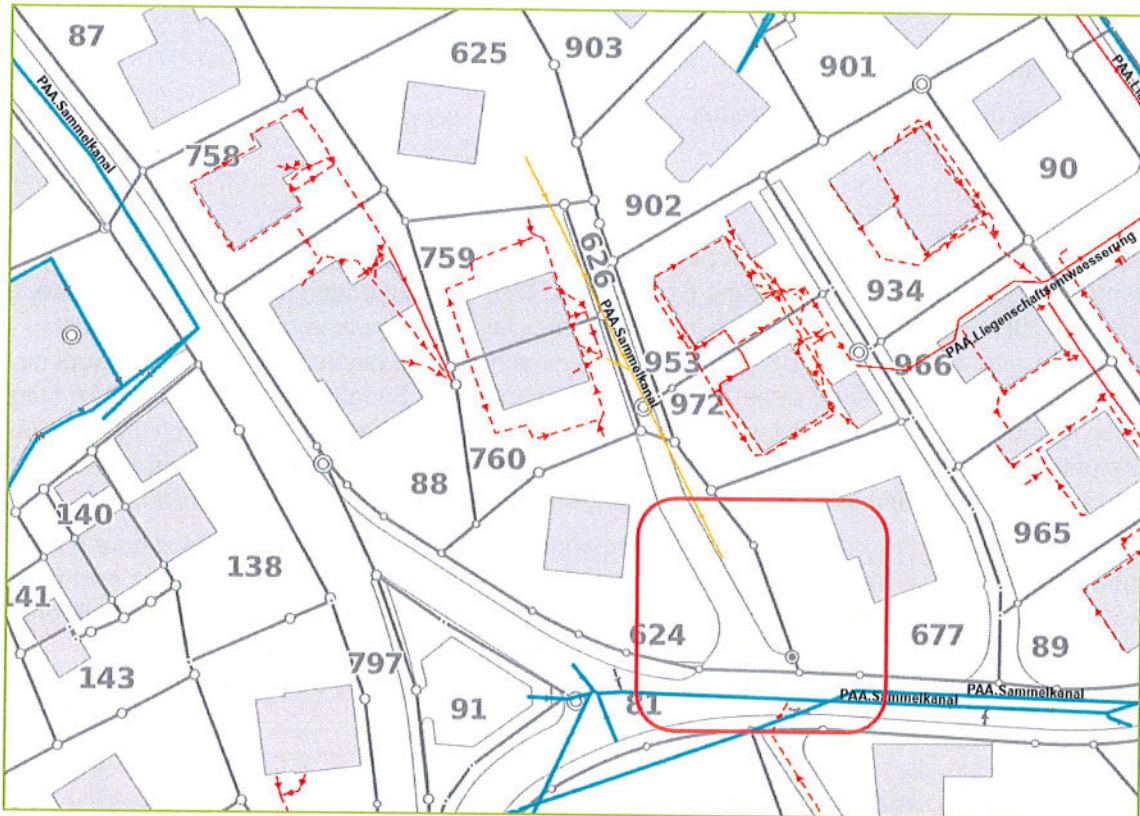
Abbildung 7 - Lücken im Leitungsnetz. Der PAA-Sammelkanal sollte mit den markierten Sammelkanälen verbunden sein.
