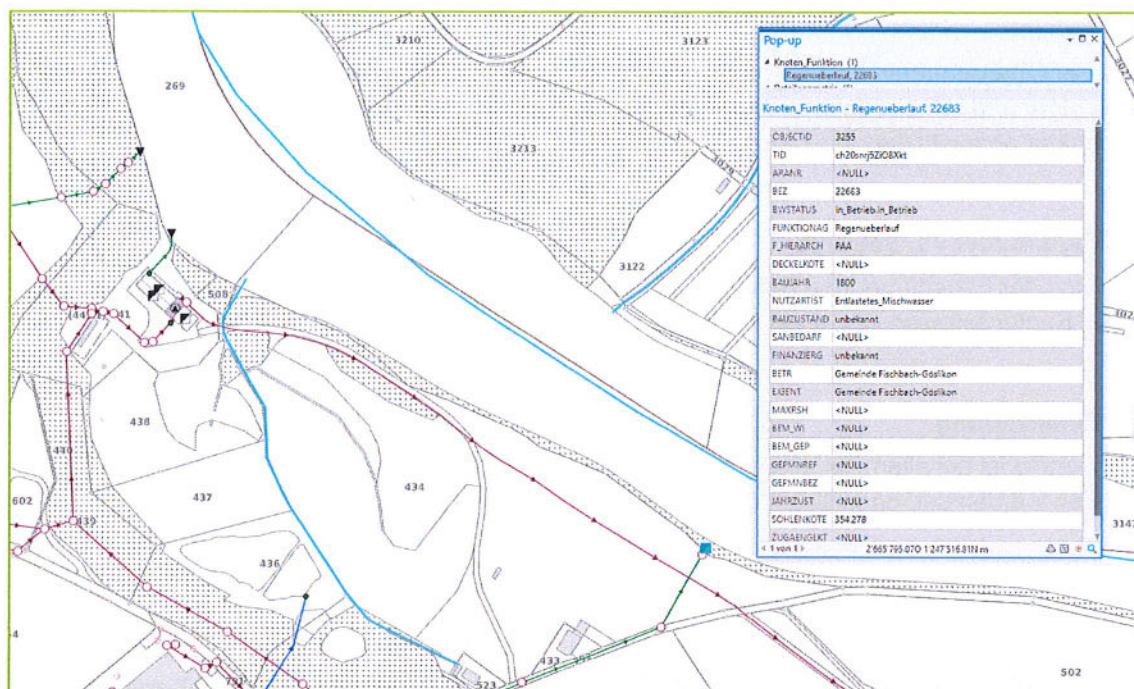
Abbildung 4 - Im linken Kartenausschnitt wurde die Schnittstelle zum Gewässer korrekt erfasst. Der markierte Knoten im rechten unteren Kartenbereich jedoch wurde als Regenüberlauf erfasst. Hier wäre ebenfalls eine Einleitstelle zu erwarten.
