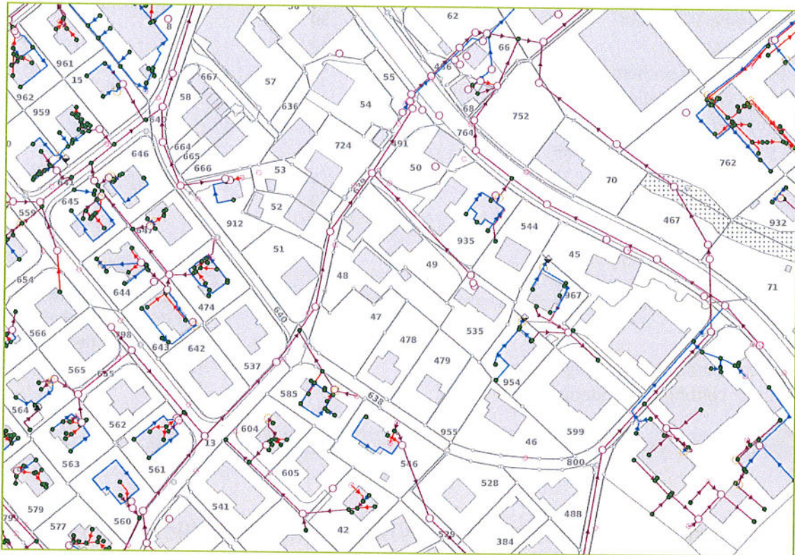
Abbildung 3 - Lücken in der Liegenschaftsentwässerung.
