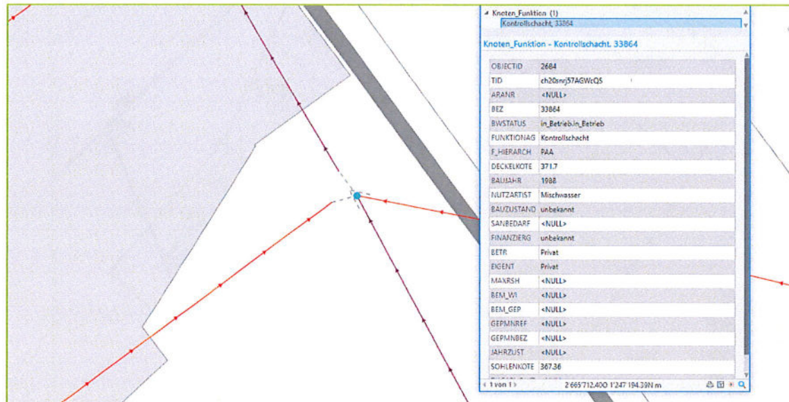
Abbildung 9 - Die Anfangs- und Endpunkte der Haltungen stimmen nicht immer mit den Knoten überein.
