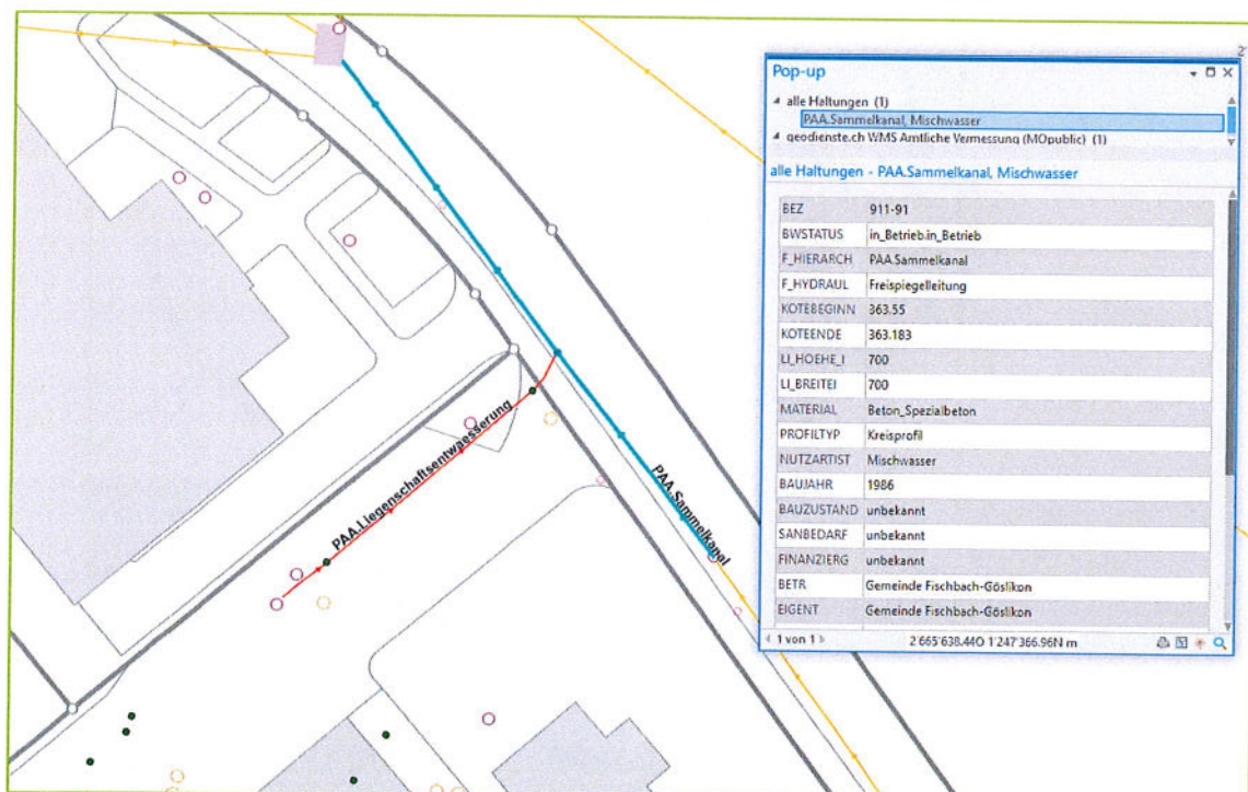
Abbildung 7 - Lücken im Leitungsnetz. Der PAA-Sammelkanal sollte mit den markierten Sammelkanälen verbunden sein.
