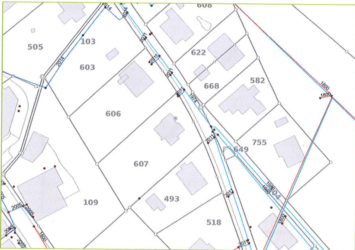
Abbildung 10 - Im Datenbestand sind Bereiche vorhanden, wo bei den Haltungen ein Baujahr erfasst wurde, aber die Knoten mit dem Baujahr 1800, also unbekannt erfasst wurden (rot eingefärbte Knoten).
