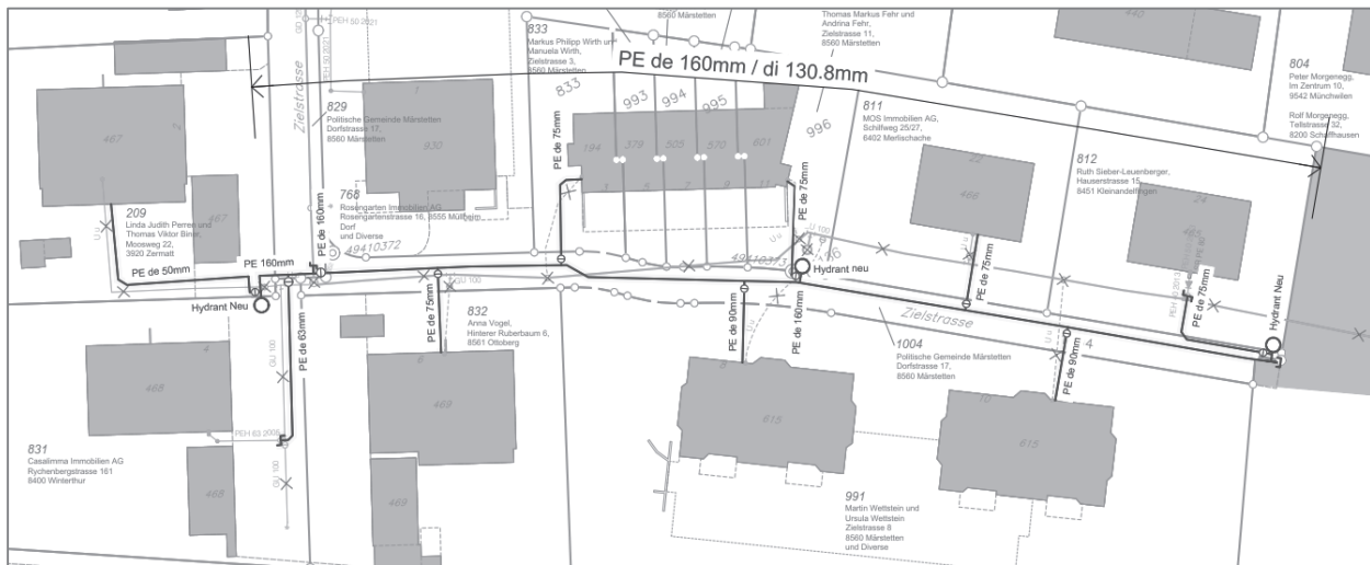
Projektplan «Wasserversorgung»
