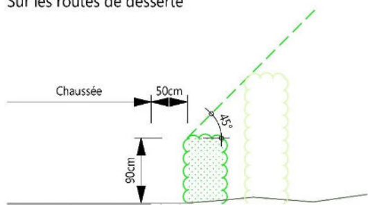
Schématisation de l'art. 138 al. 1 point a) "sur les routes de desserte" et al. 2
