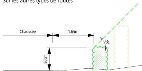
Schématisation de l'art. 138 al. 1 point b) "sur les autres types de routes" et al. 2
