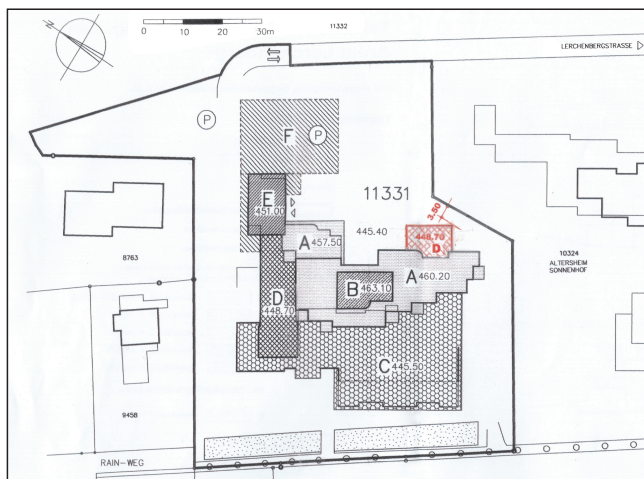
Situation mit erweitertem Baubereich D (Änderung: rot)
