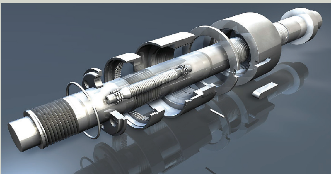
Satelliten-Rollspindel von Ziegler.
