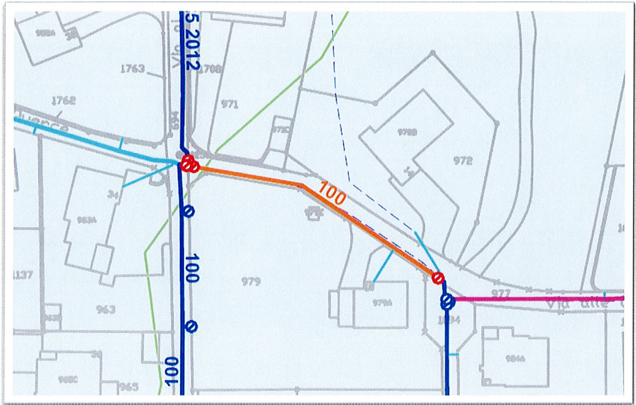
Condotte acqua potabili interventi calcolo idraulico tappa 3 (arancione) (PGA 2014)
