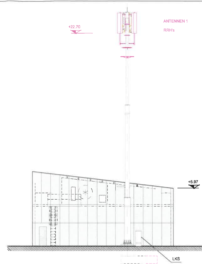
OSTANSICHT 1:200
