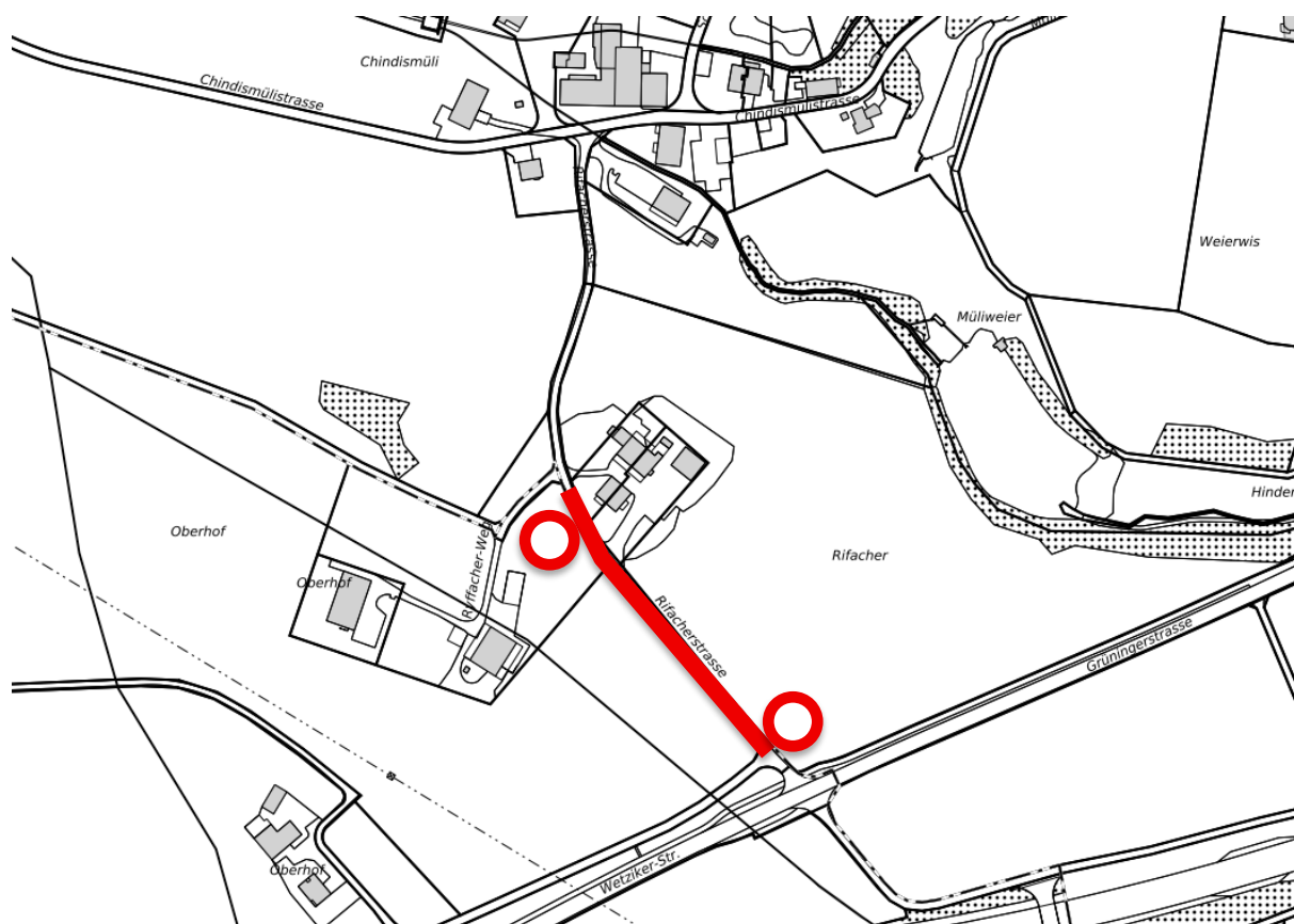
Lichtraumprofil in der Höhe h: 4,5 m
