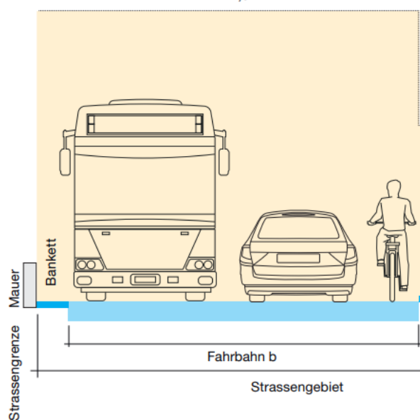
Lichtraumprofil in der Höhe h: 4,5 m
