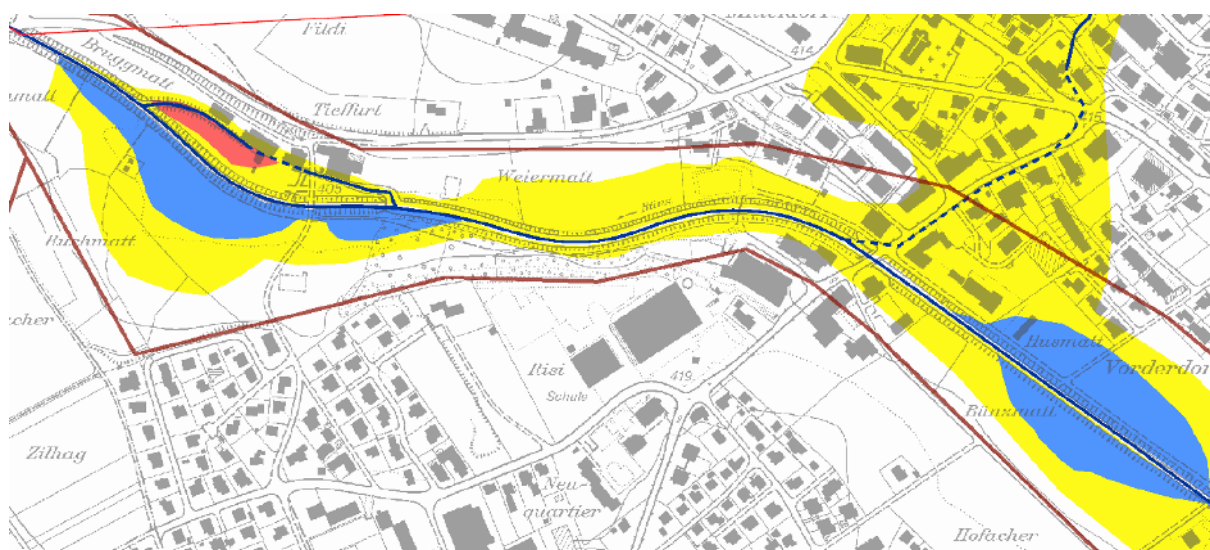
Abb. 9: Ausschnitt aus der Gefahrenkarte Hochwasser im Ist-Zustand; rot: erhebliche Gefährdung, blau: mittlere Gefährdung, gelb: geringe Gefährdung [27].
