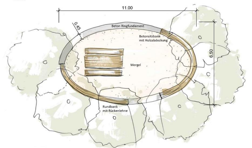
Situation Sitzplatz M 1:100
