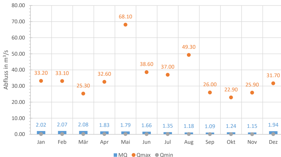
Abb. 5: Jahreszeitliche Verteilung der Abflüsse am Pegel FG_0332 unter Angabe des Mittleren Abflusses (MQ) und des jeweils höchsten ( Q_{max} ) bzw. niedrigsten Wertes ( Q_{min} ) pro Monat in der gesamten Auswertungsperiode von 1977-2019.
