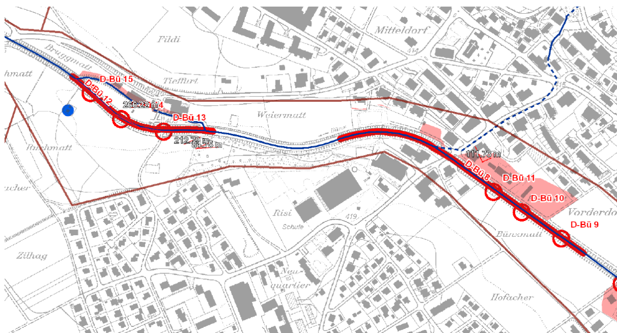
Abb. 10: Ausschnitt aus der Gefahrenkarte Hochwasser Schutzdefizite; rote Flächen, blaue Punkte: Schutzdefizite, rote Linien und Kreise: Austrittsstellen.
