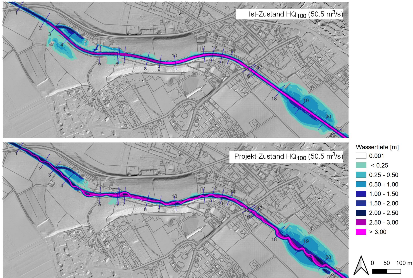
Abb. 19: Wassertiefen bei einem hundertjährigen Hochwasser HQ 100 im Ist- und im Projektzustand.
