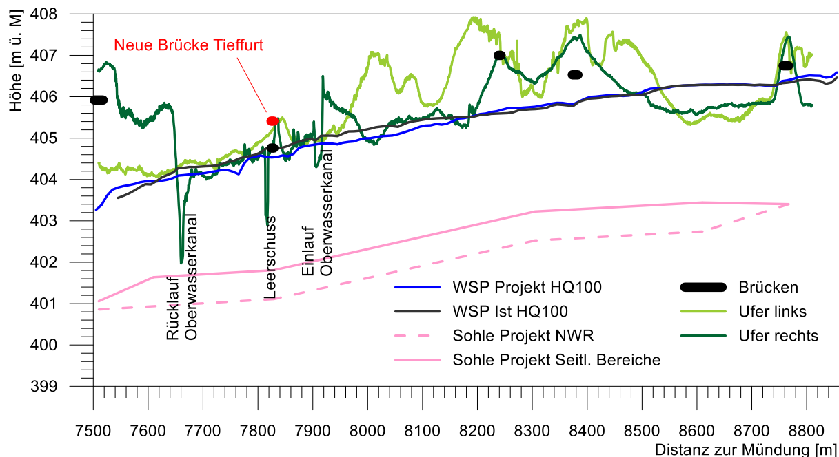
Abb. 16: Längsprofil der Wasserspiegellagen bei einem hundertjährigen Hochwasser HQ_{100} im Ist- und im Projektzustand.
