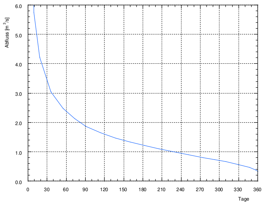
Abb. 4: Dauerkurve der Überschreitungstage der Bünz am Pegel FG 0332. Ausgewertete Periode 1977-2019.
