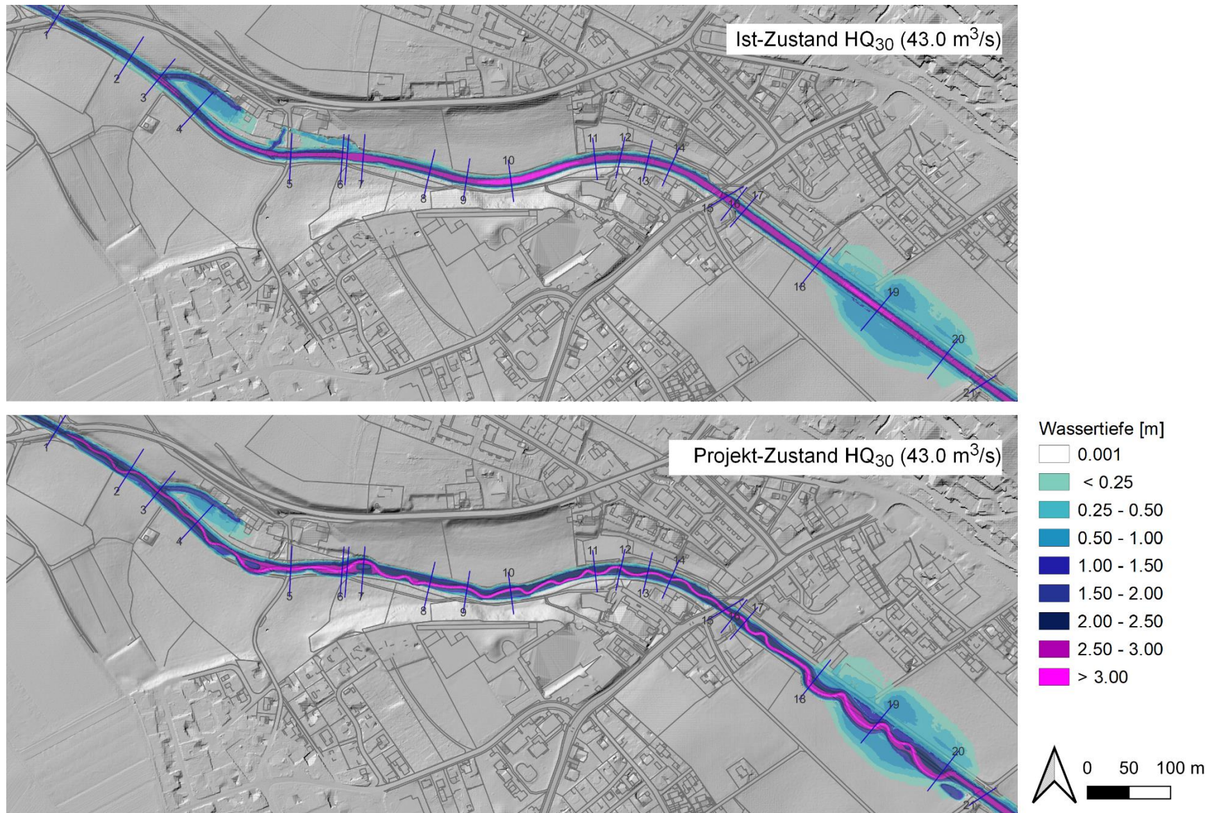
Abb. 18: Wassertiefen bei einem dreissigjährigen Hochwasser HQ 30 im Ist- und im Projektzustand.
