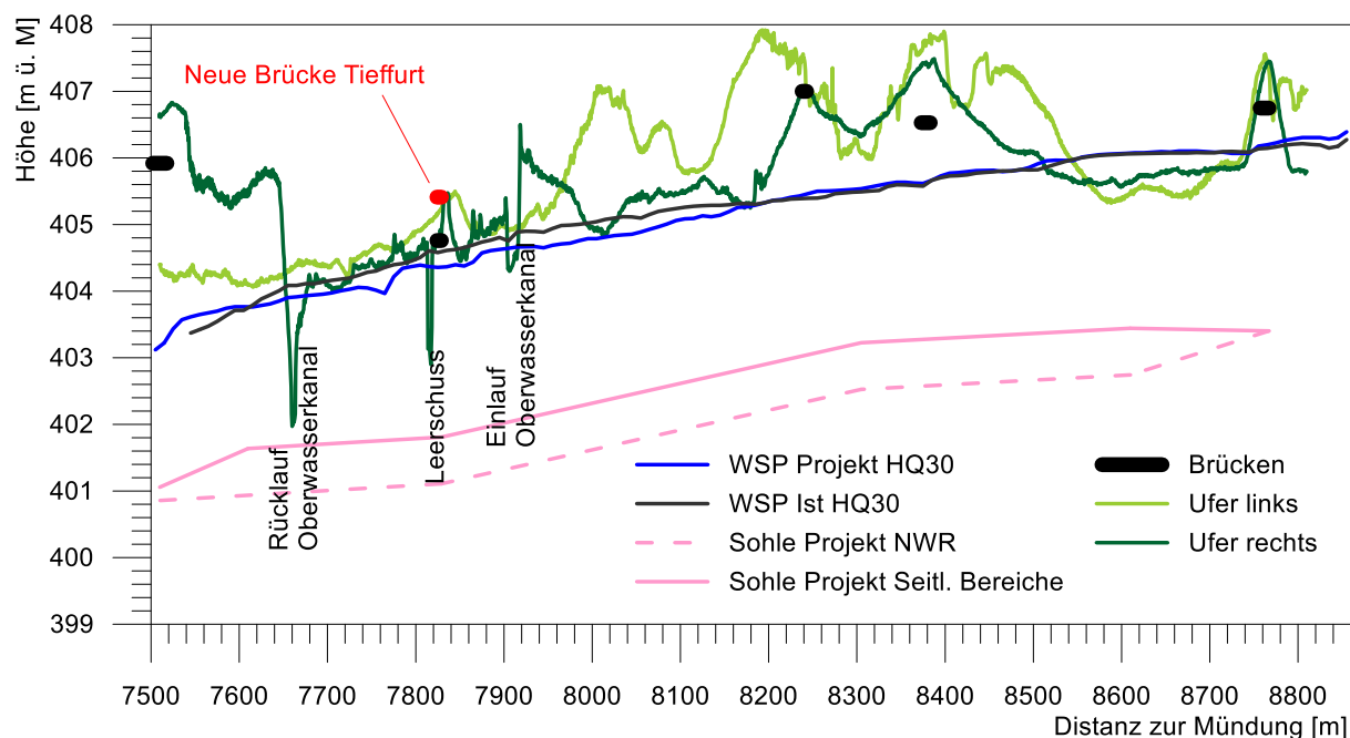
Abb. 15: Längsprofil der Wasserspiegellagen bei einem dreissigjährigen Hochwasser HQ_{30} im Ist- und im Projektzustand.
