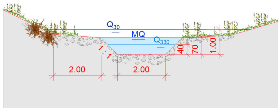
Abb. 13: Normprofil zur Veranschaulichung des Gerinnequerschnitts und der korrespondierenden Wasserspiegel.
