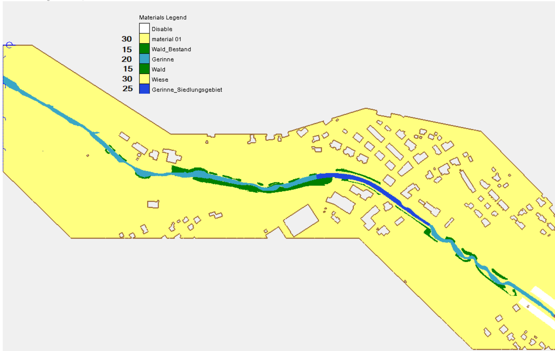
Abb. 17: Verwendete Rauigkeitsbeiwerte in m^{1/3}/s im Projektzustand.
