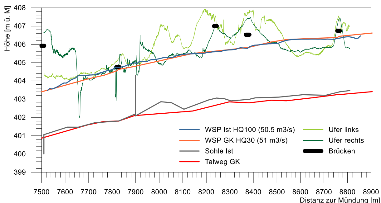
Abb. 14: Längenprofil der Wasserspiegellagen der Gefahrenkarte im Vergleich mit dem Ist-Zustand des 2d-Modells.
