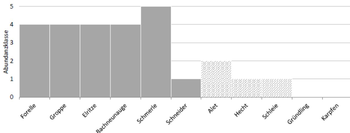
Abb. 12: Vermutete historische Referenz der Fische für die Bünz in Hendschiken. Grau: für Bachforellenregion typisch, schraffiert: für Bachforellenregion atypisch).
