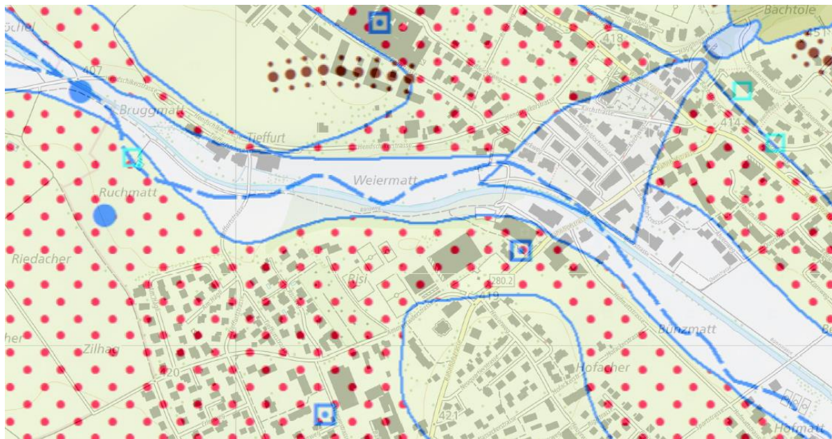
Abb. 3: Ausschnitt aus dem Geologischen Vektordatensatz GeoCover [24].
