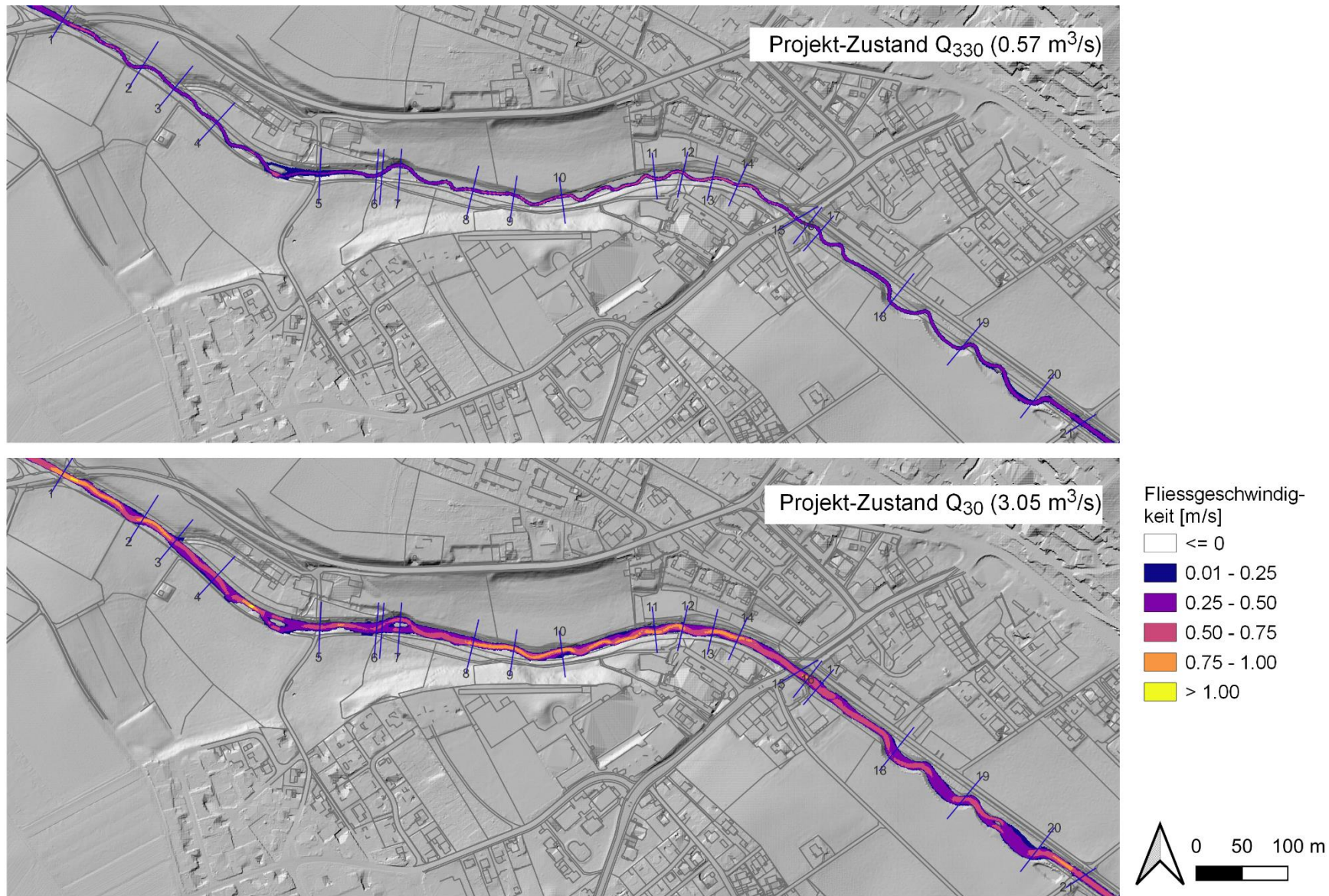
Abb. 21: Fließgeschwindigkeit bei Q_{330} und Q_{30} im Projektzustand.
