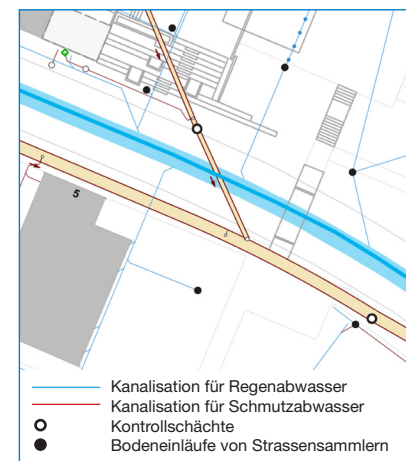
Der Katasterplan gibt Auskunft über die Lage der Schmutz- und Regenabwasserkanäle.
