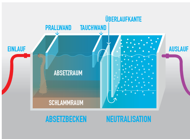
Korrekt installiertes Absetzbecken.
