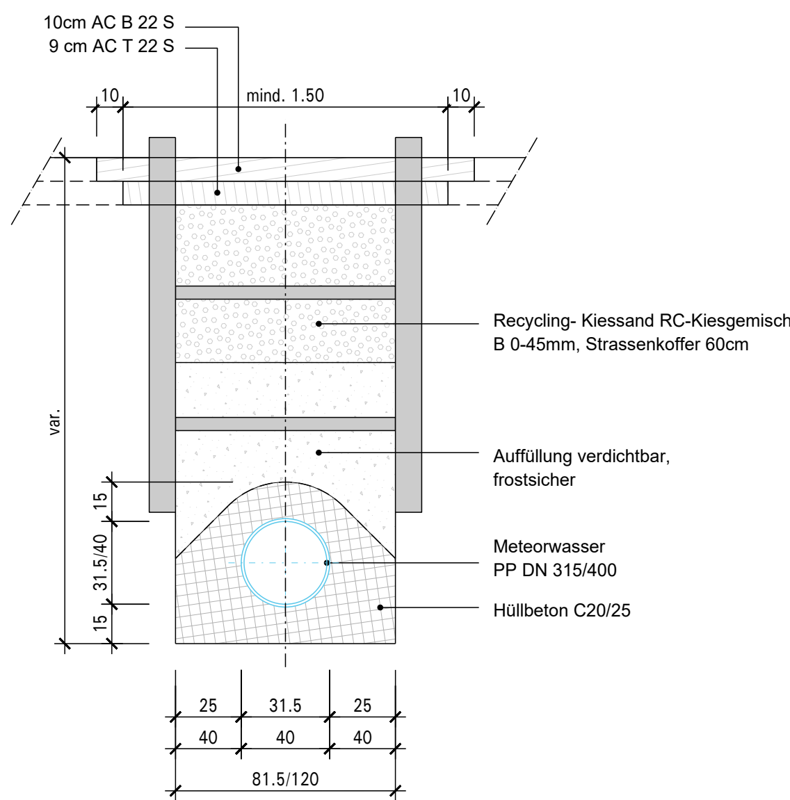
Grabennormalprofil 1:20
