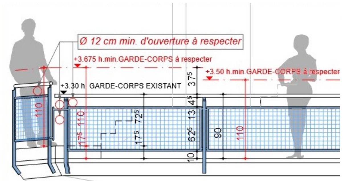
Fig. 5 - Hauteurs garde-corps actuel / à respecter
