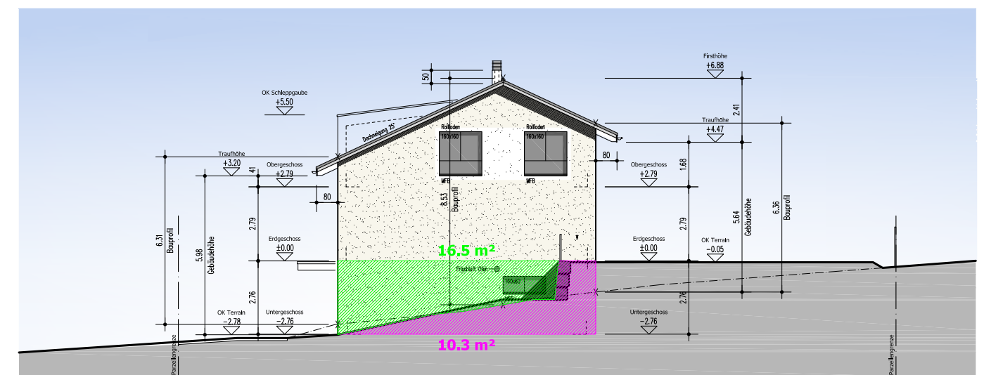
Nordwestfassade
