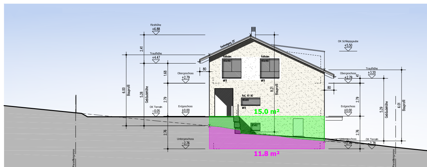
Südostfassade
