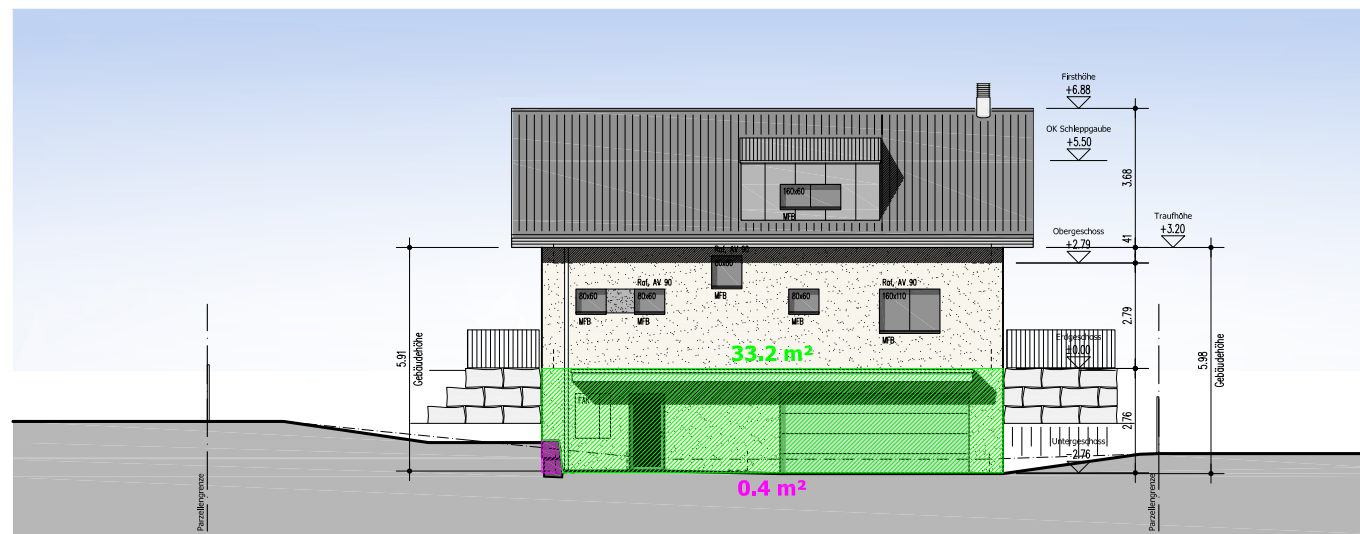
Nordostfassade
