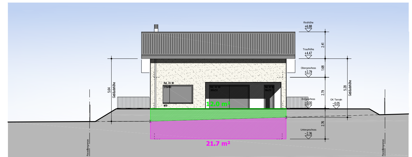
Südwestfassade
