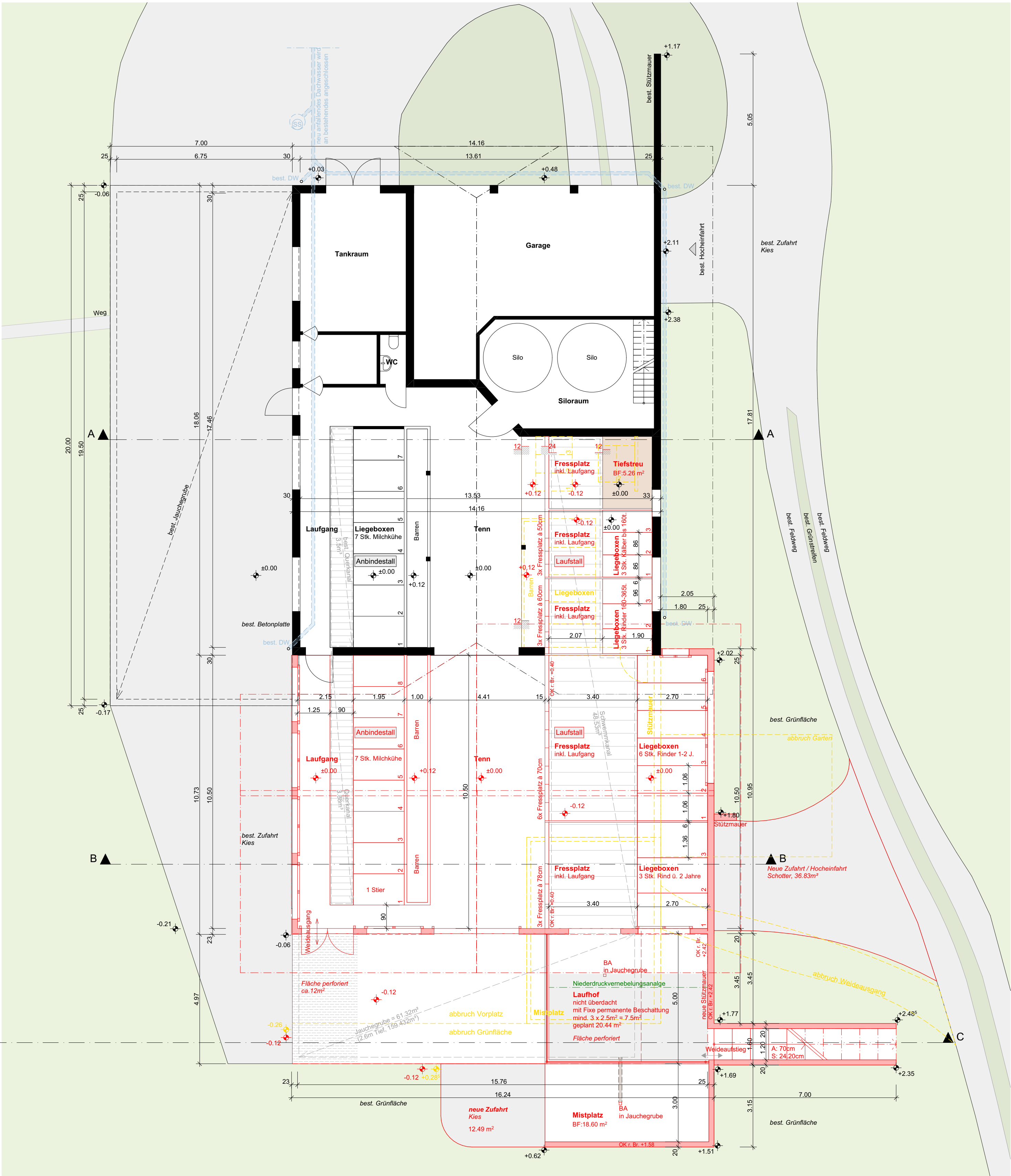
Erdgeschoss
