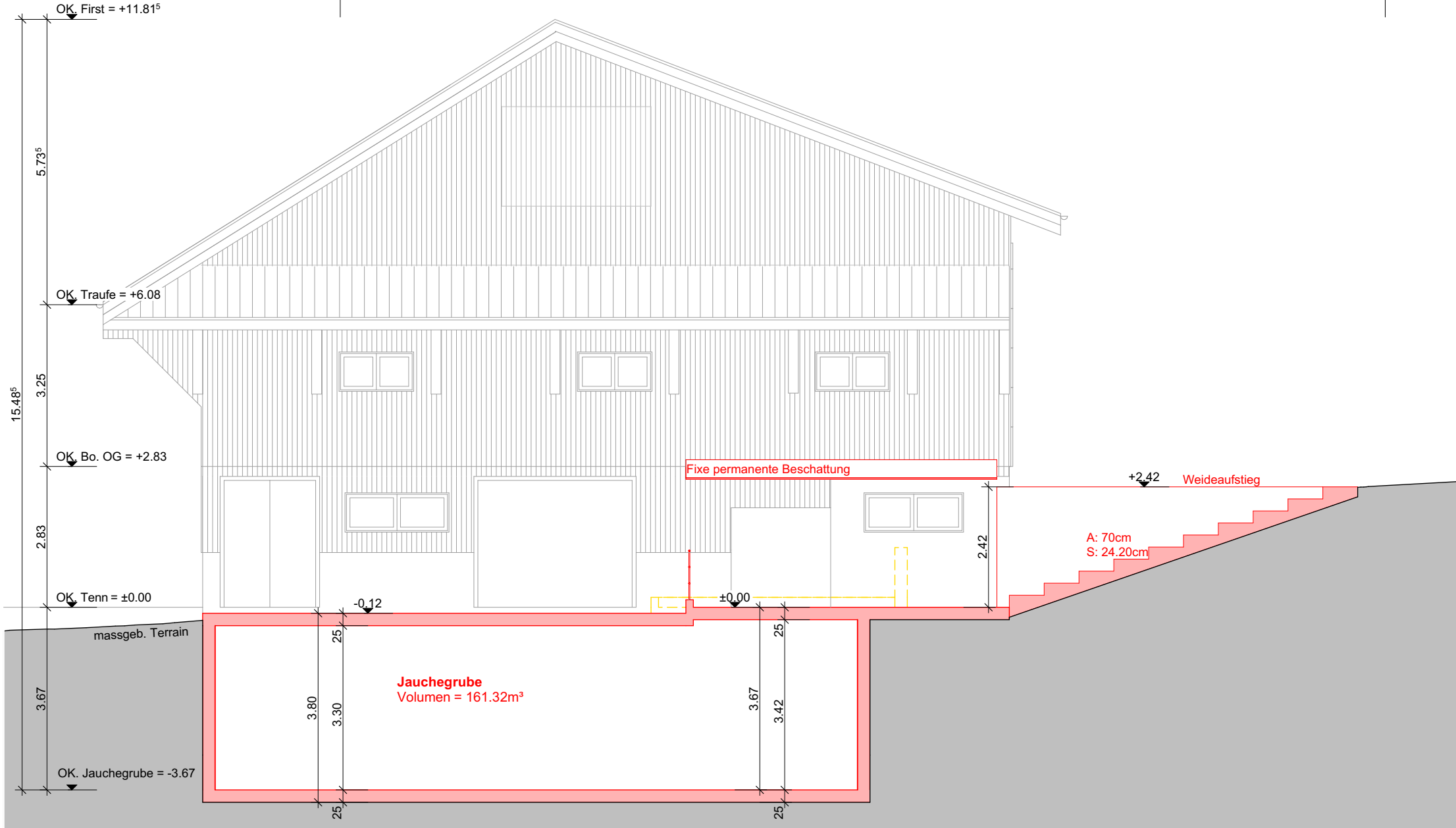
Schnitt C-C
