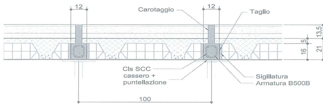
Immagine: intervento tipo di rinforzo
