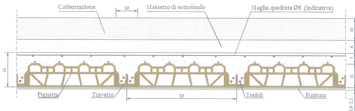
Immagine: soletta tipo di copertura 1. piano
