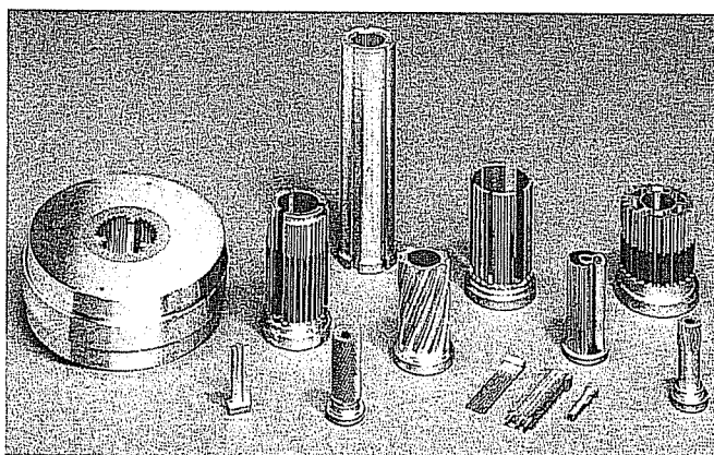
Diverse Formwerkzeuge
