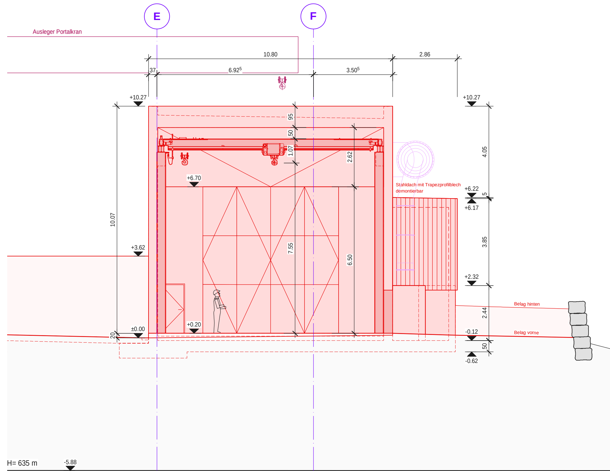
Südostfassade 1:100
