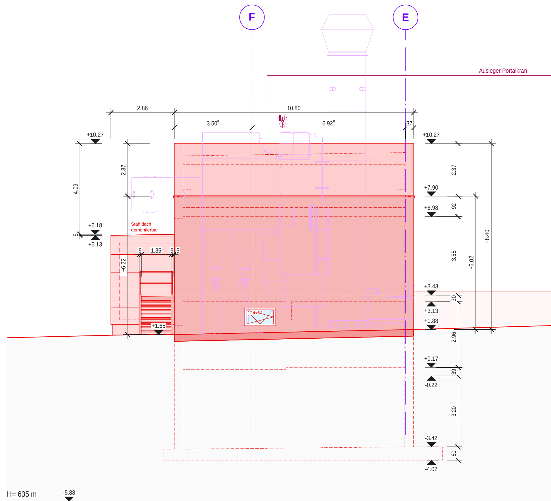
Nordwestfassade 1:100
