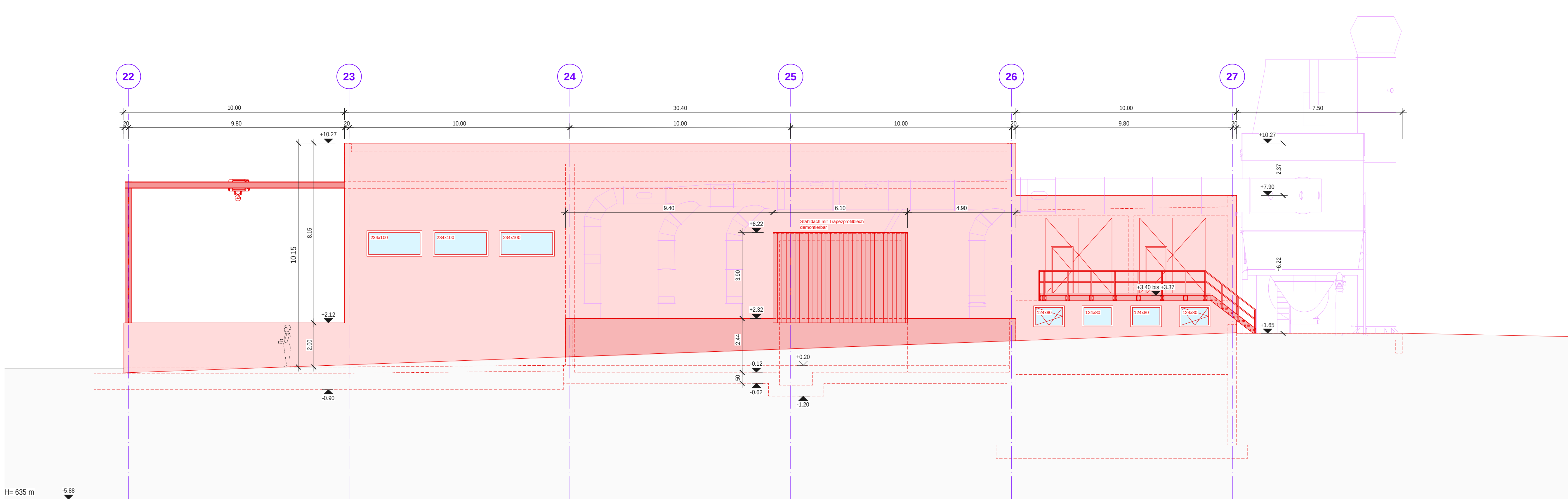
Nordostfassade 1:100
