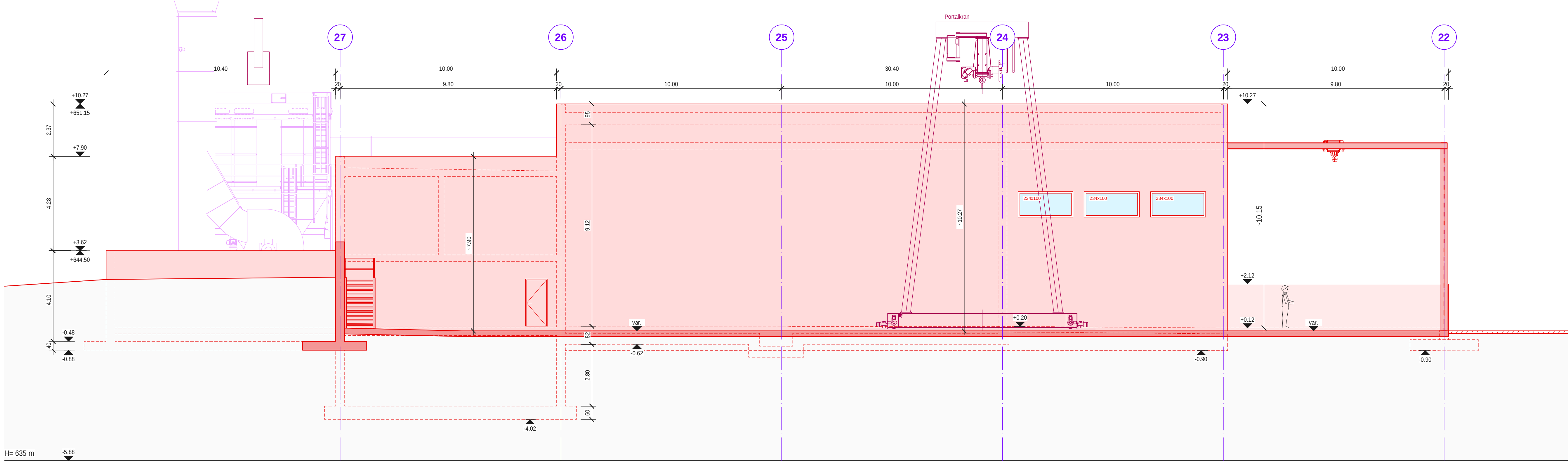
Südwestfassade 1:100
