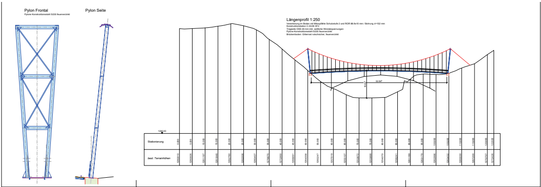
Pilons (vista frontala e da la vart) e profil longitudinal
