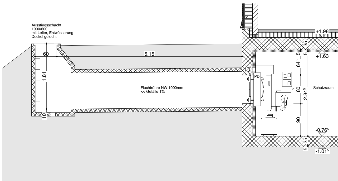
SCHNITT FLUCHTRÖHRE | MST. 1:50
