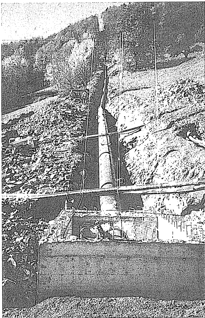
DRUCKLEITUNG VORDERBERG-ALTENDORF (Aufnahme November 1986)
