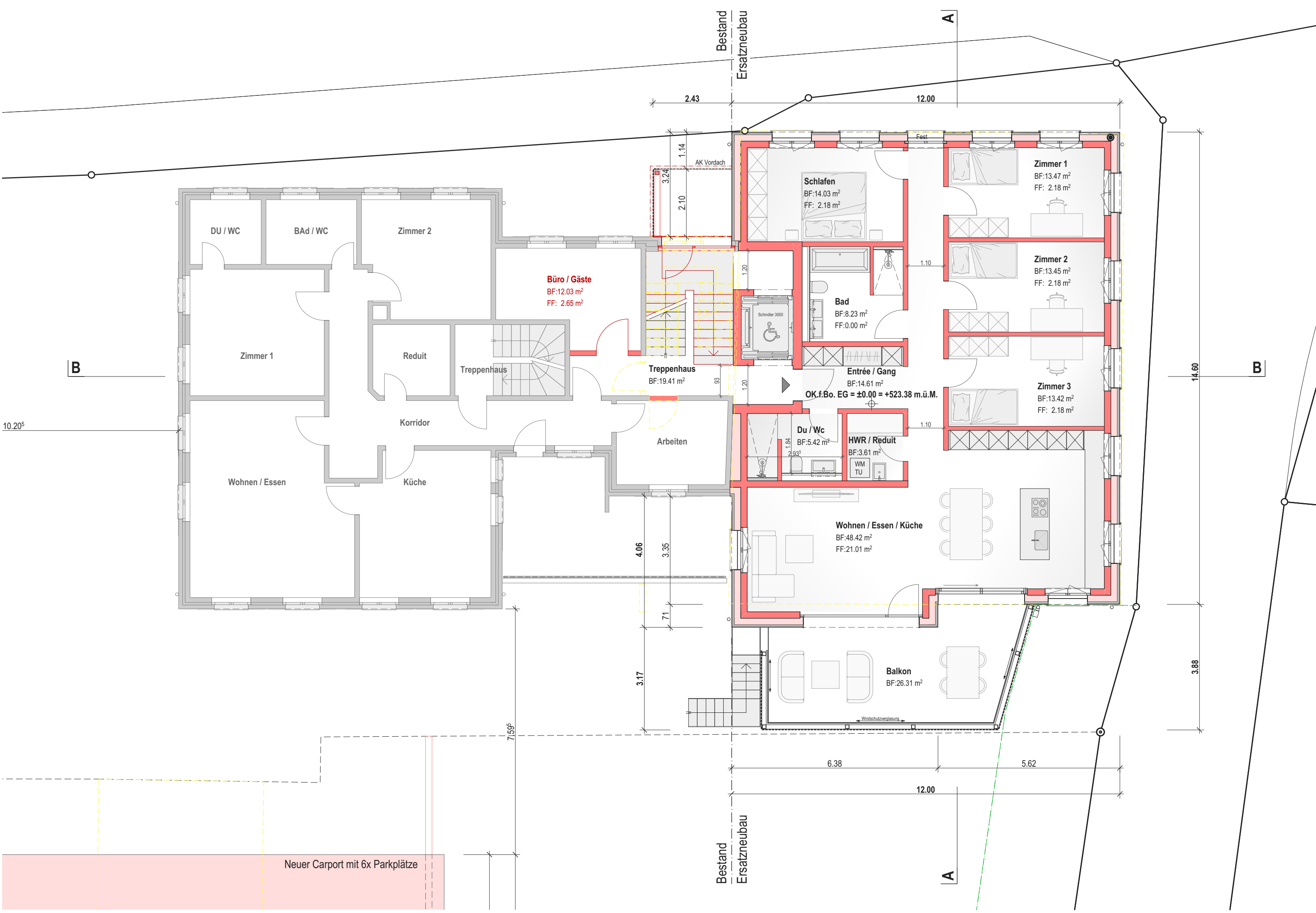
Erdgeschoss | Mst. 1:100
