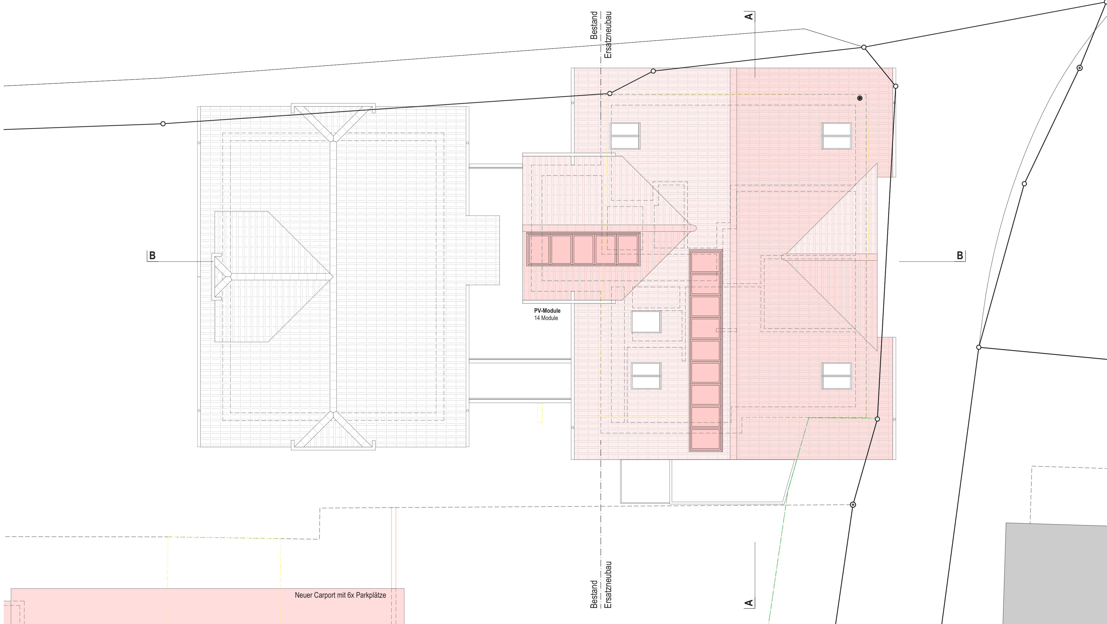
Dachaufsicht | Mst. 1:100
