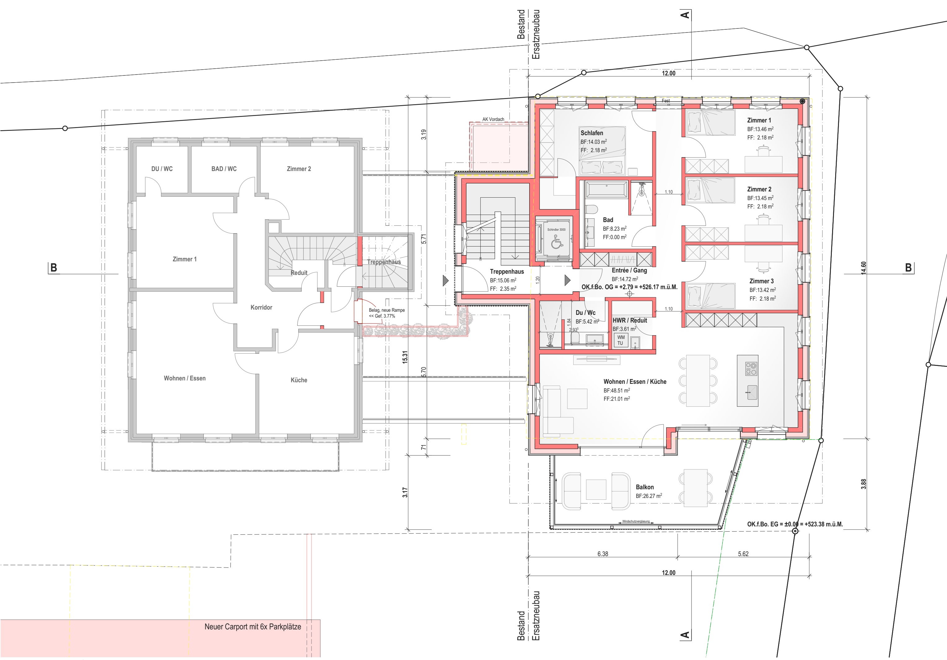
Obergeschoss | Mst. 1:100
