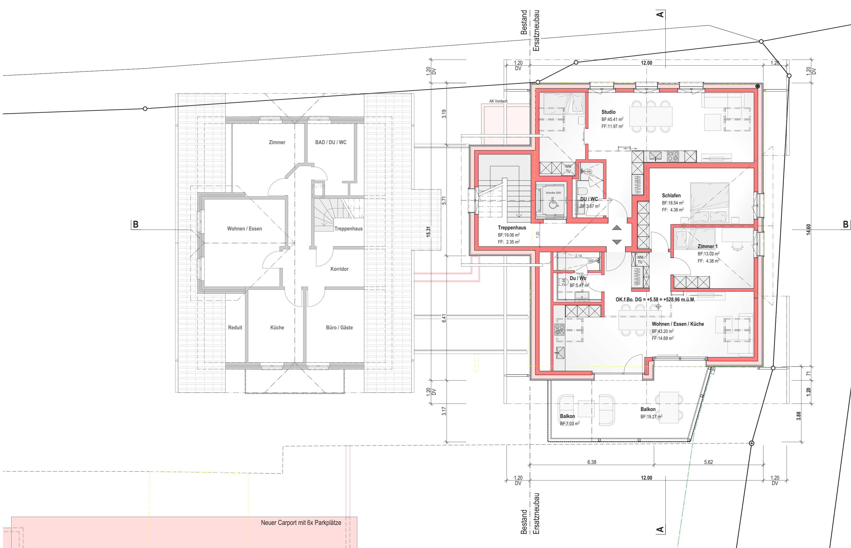
Dachgeschoss | Mst. 1:100
