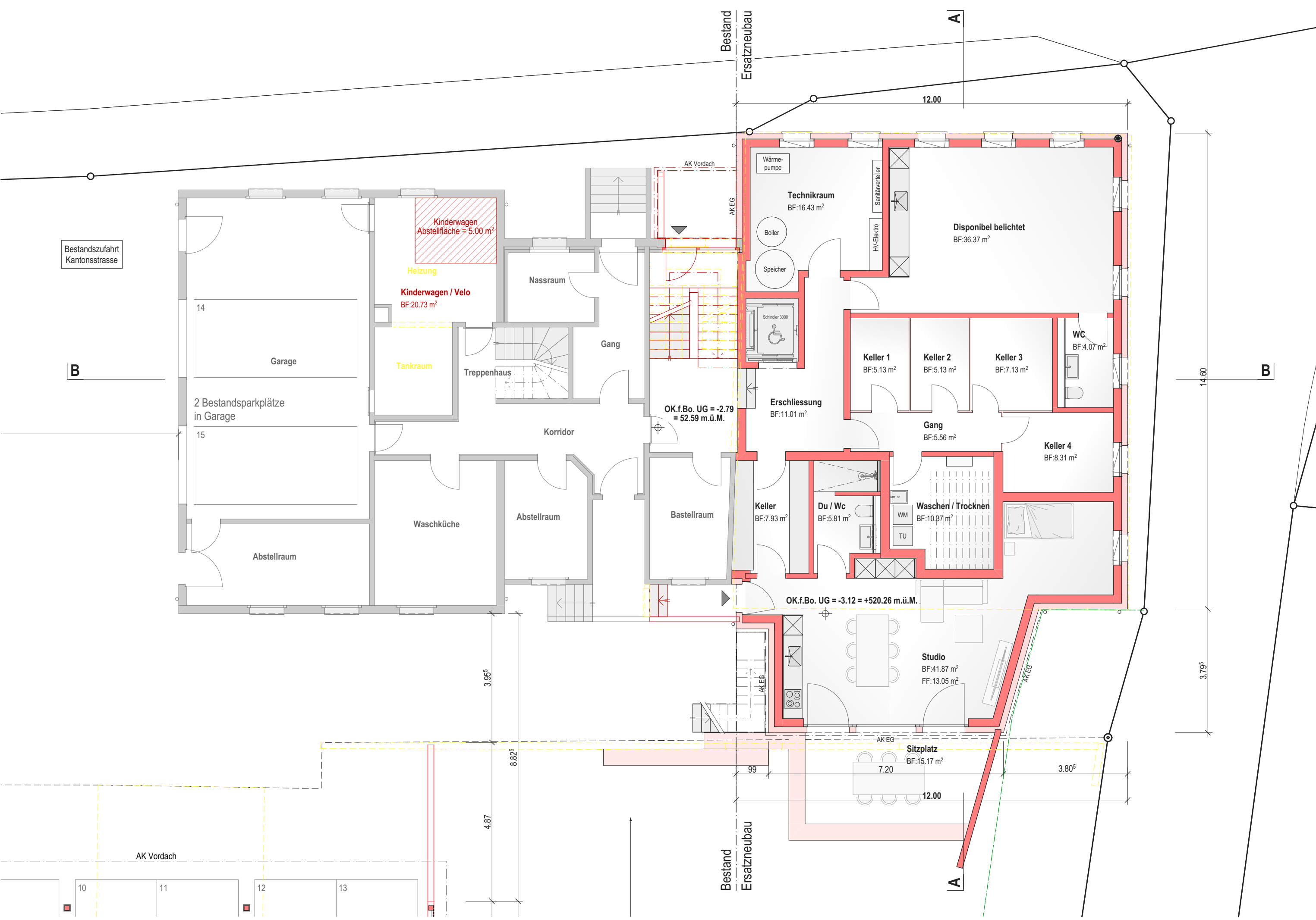
Untergeschoss | Mst. 1:100
