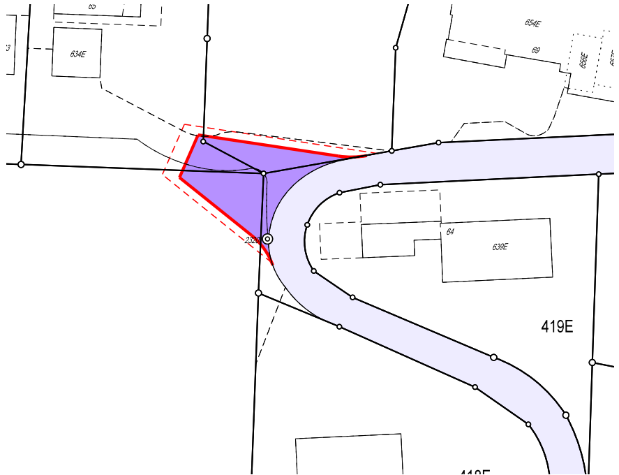
■ An der Sonnenbergstrasse soll ein Wendehammer realisiert werden
