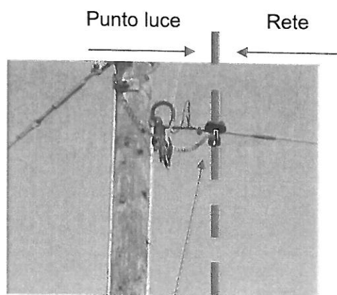
Morsetti (esterni)
