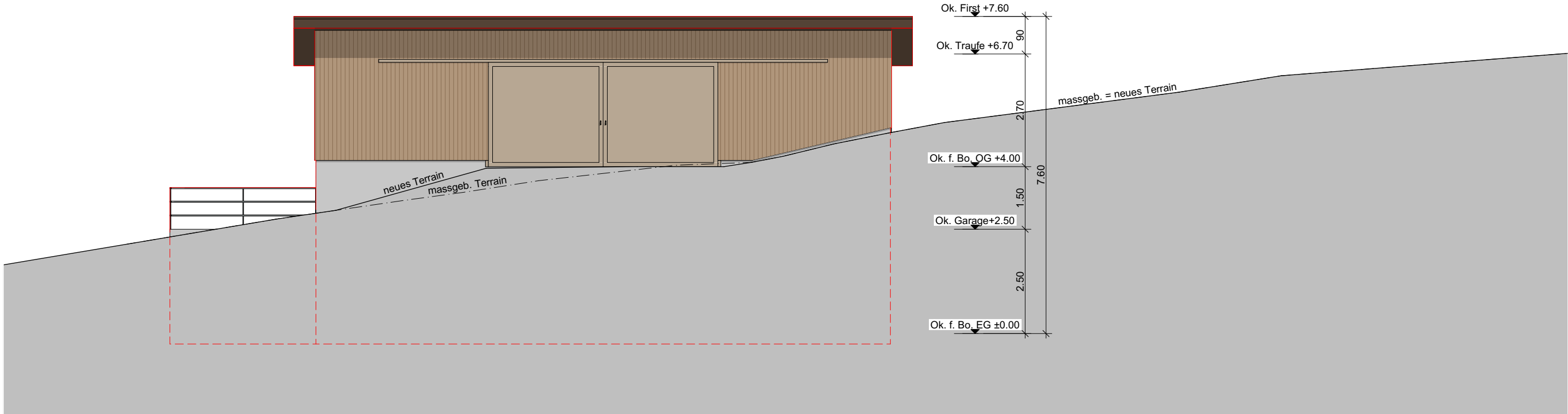
Südfassade
