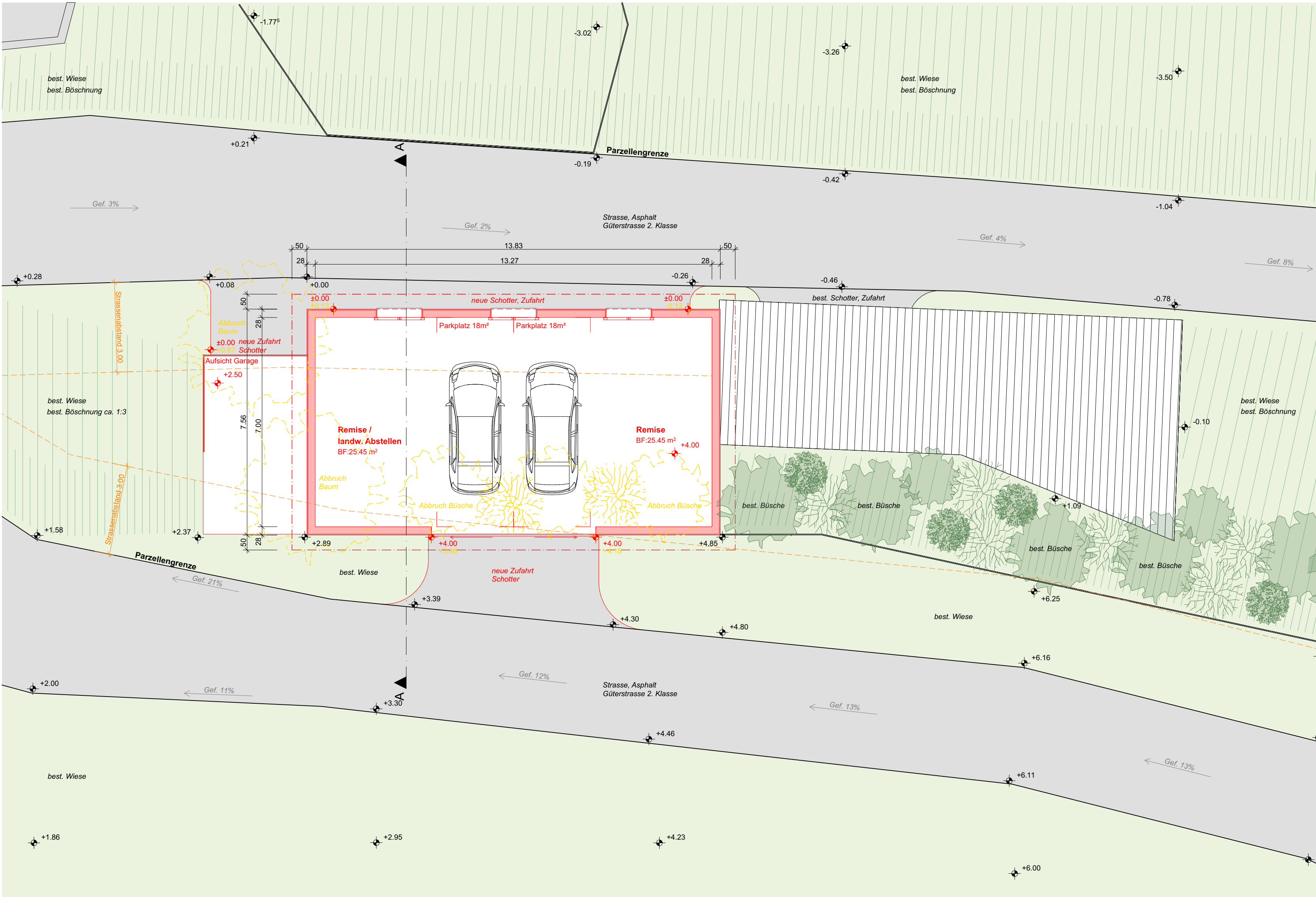
Obergeschoss / Umgebung
