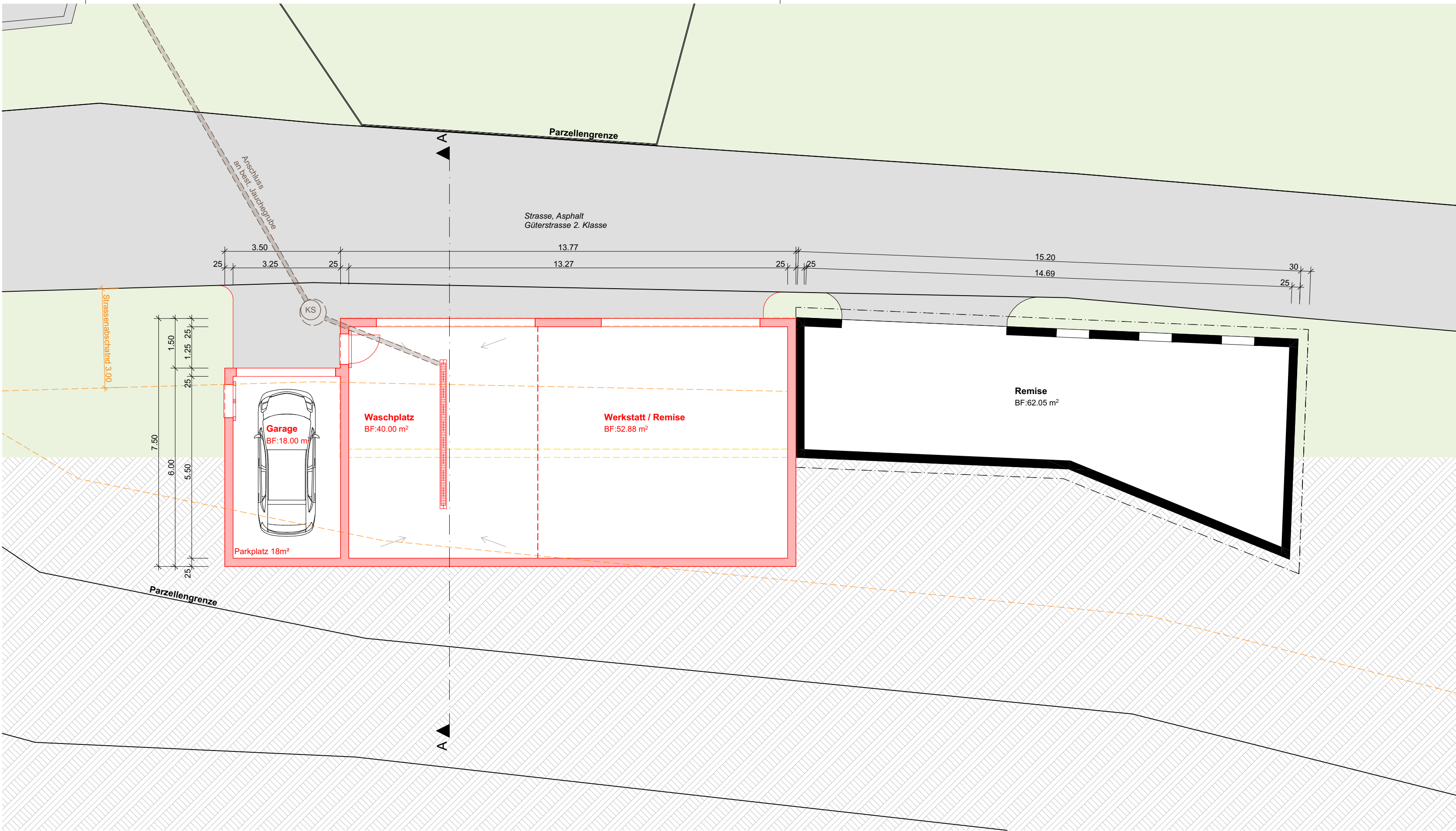
Erdgeschoss
