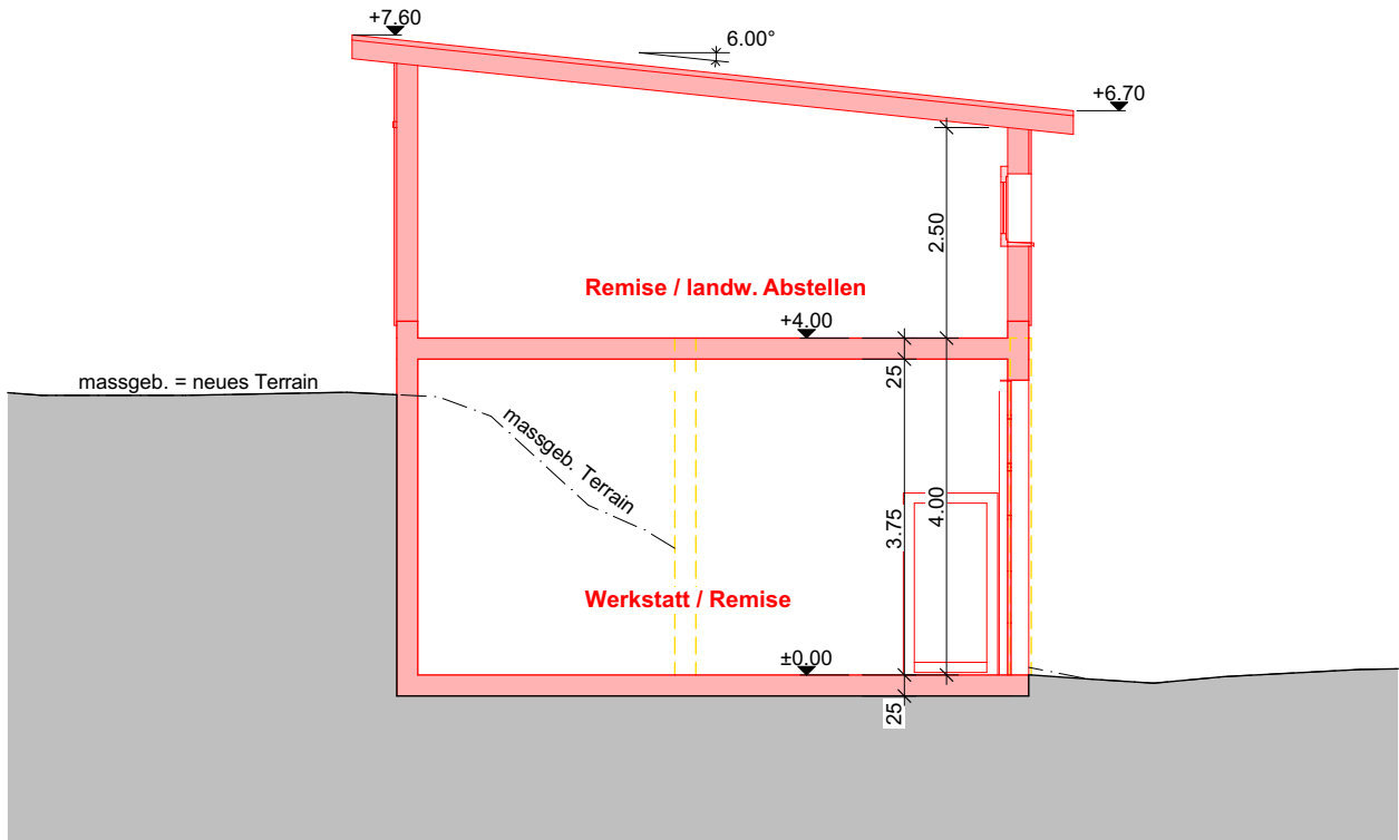
Schnitt A-A
