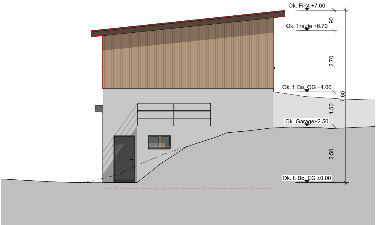
Westfassade
