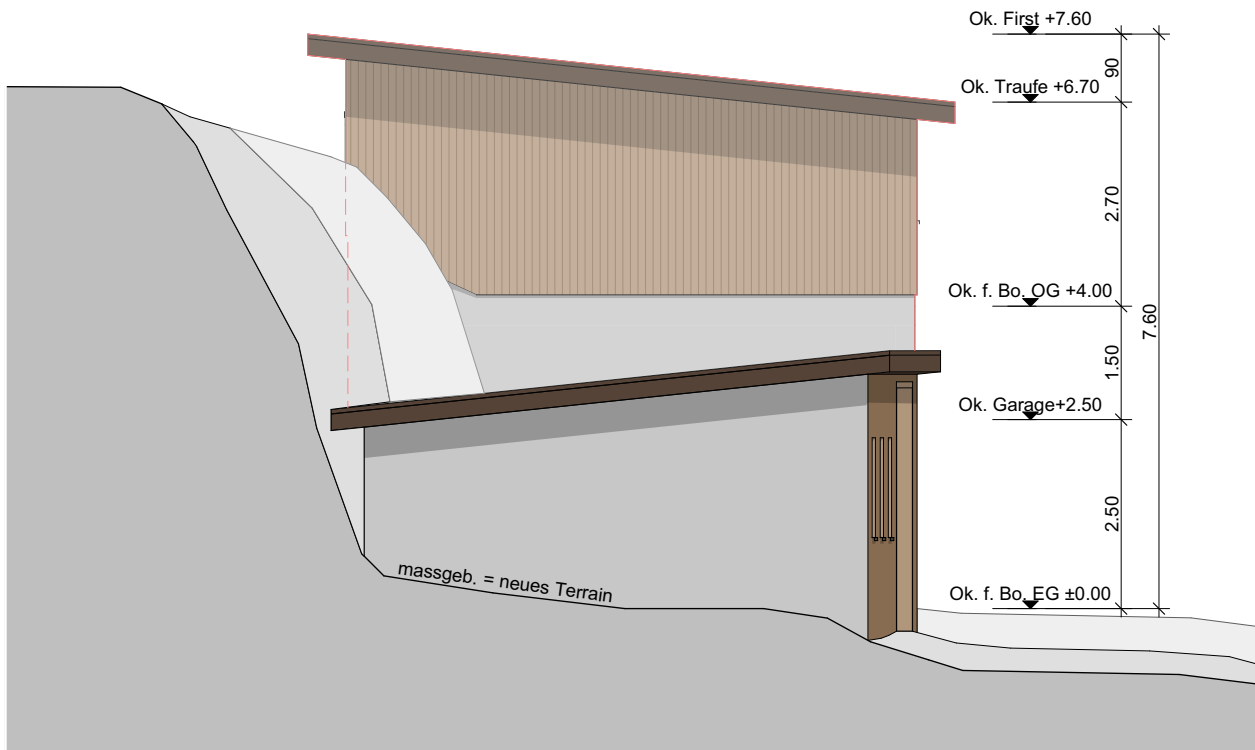
Ostfassade
