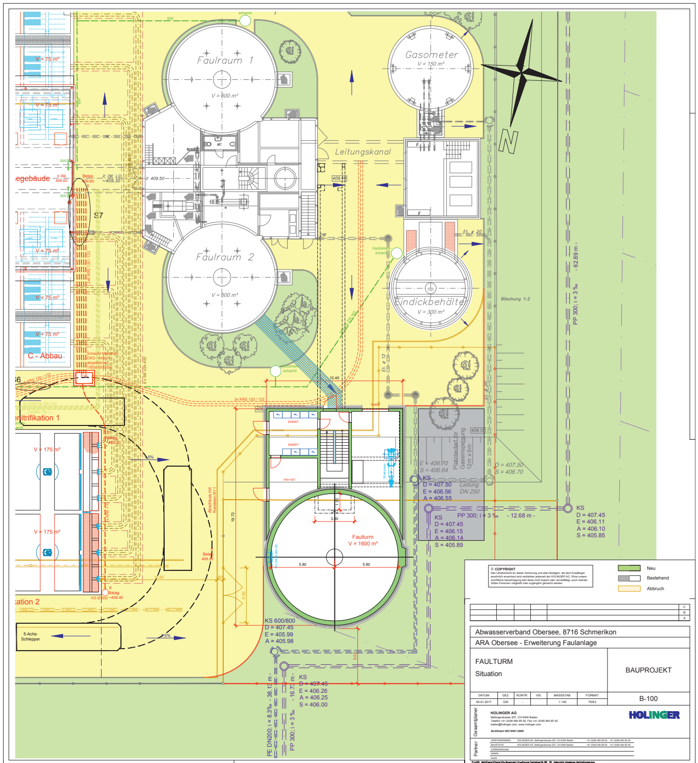
Situationsplan der erweiterten Faulanlage
