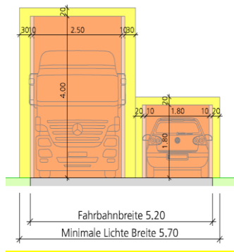
Begegnung Lastwagen / Personenwagen Geschwindigkeit 30 km/h, gemäss SN640201, 1992
