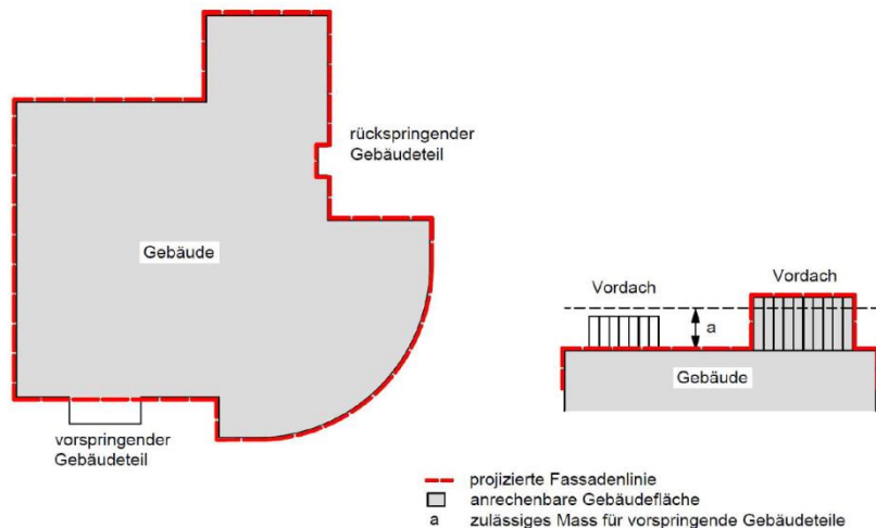
Abbildung 20 Überbauungsziffer (Figur 15 KBV), a = 1.2\text{m}
