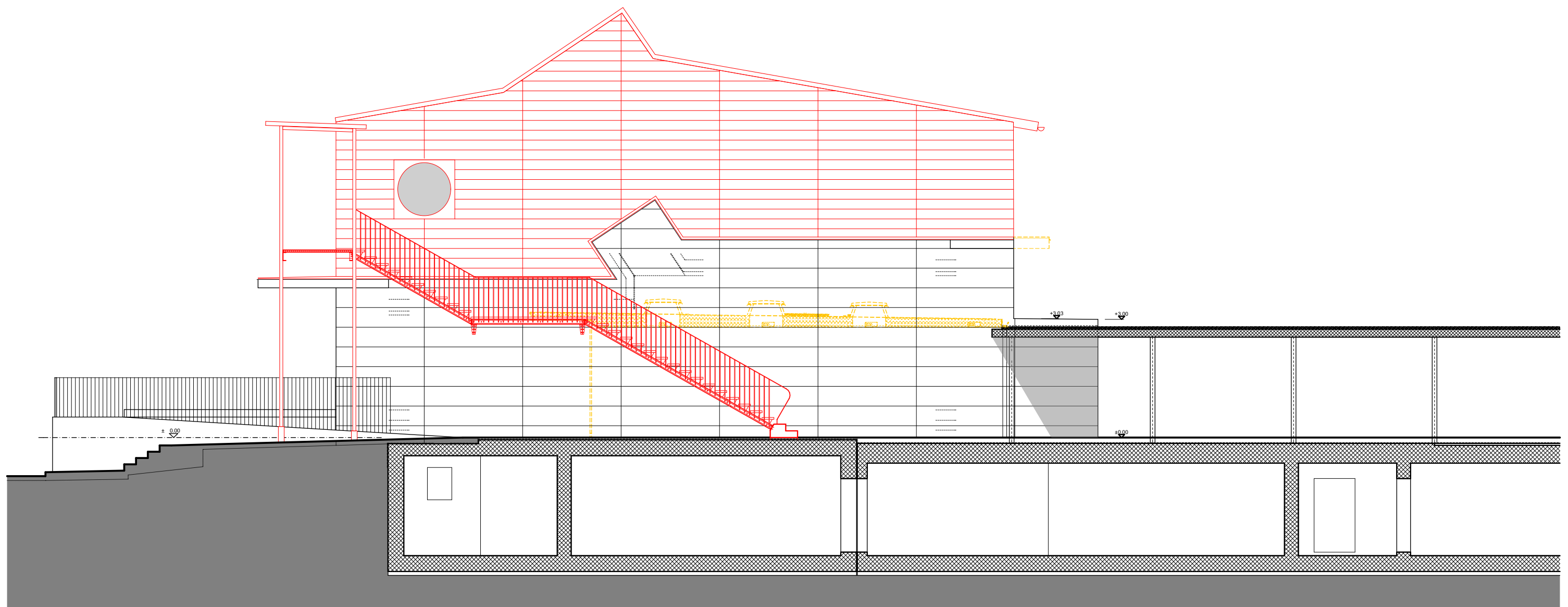
Westfassade
