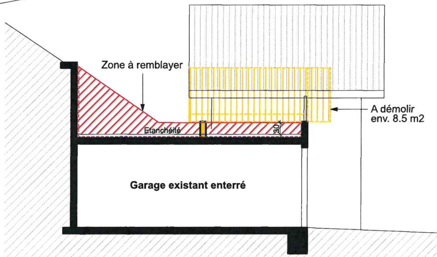
Coupe Y-Y 1/100
