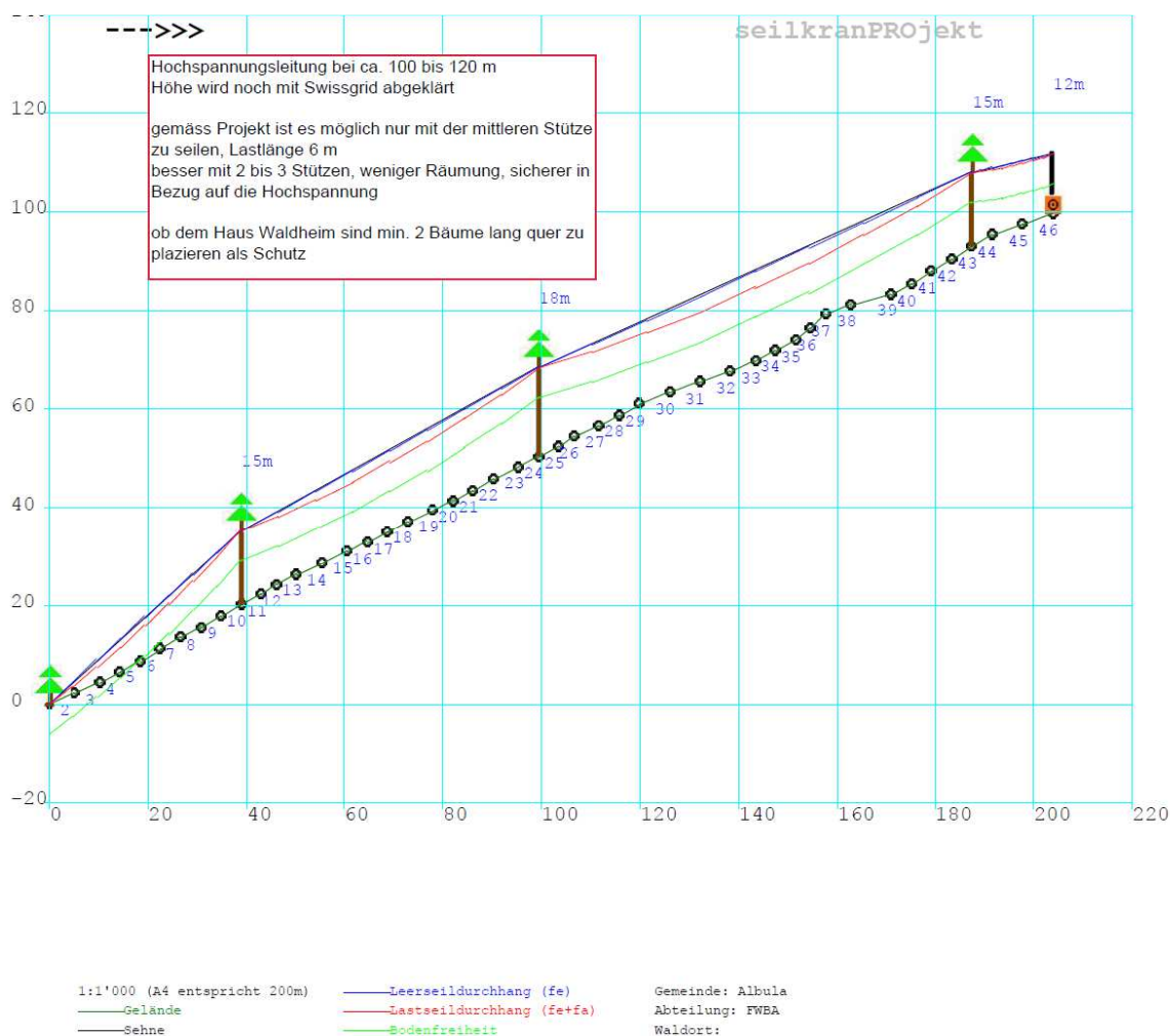
Detailprojekt der ersten Seillinie mit Bergtransport
