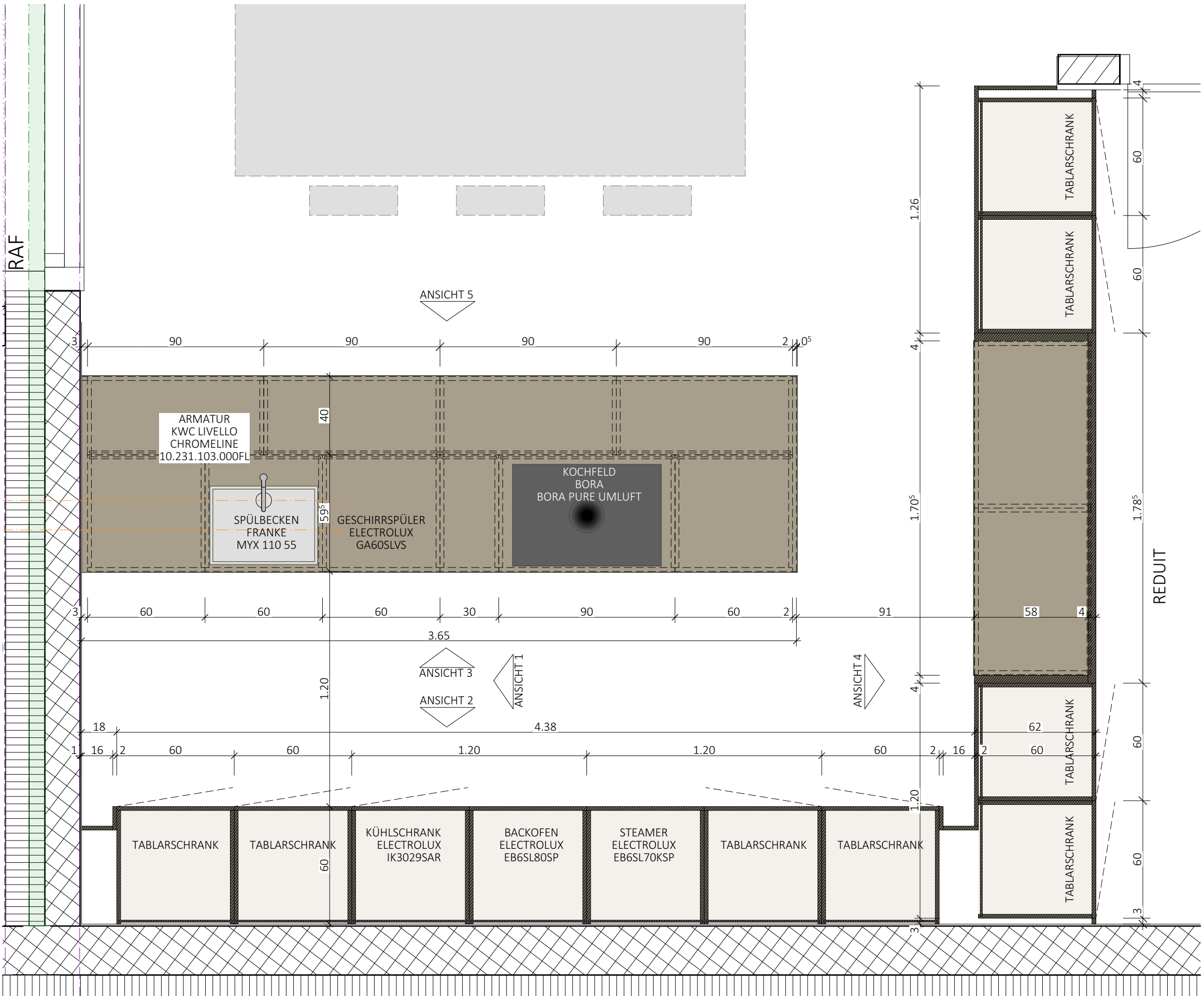
GRUNDRISS KÜCHE EG
