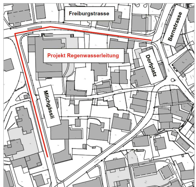
Schemaskizze der neuen Regenwasserleitung.
