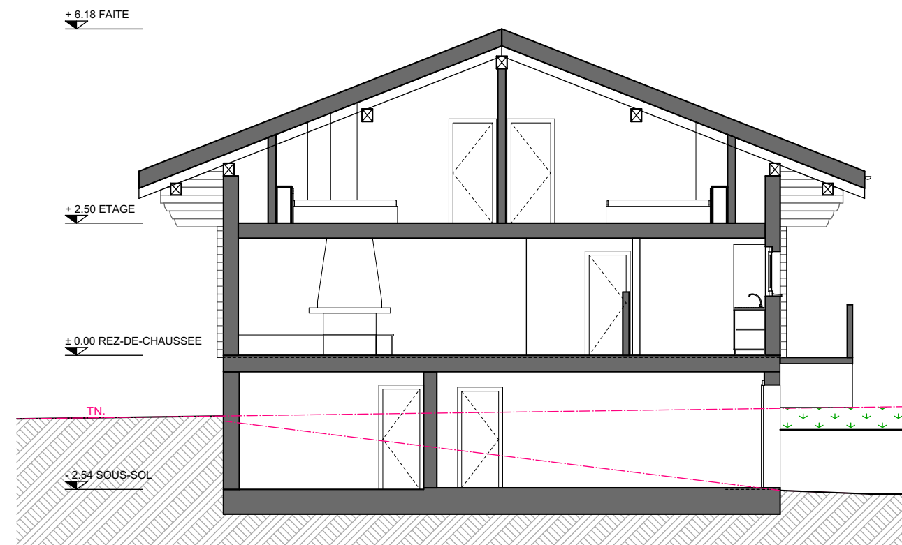
COUPE A-A
