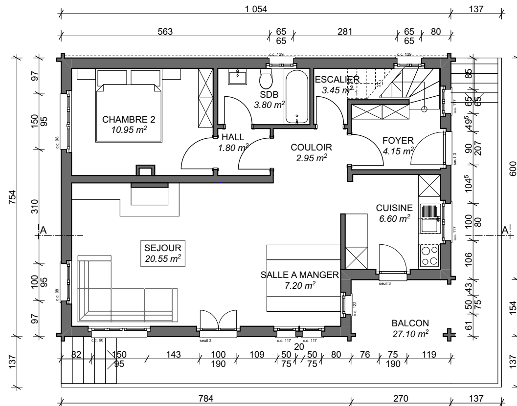
REZ SUPERIEUR
